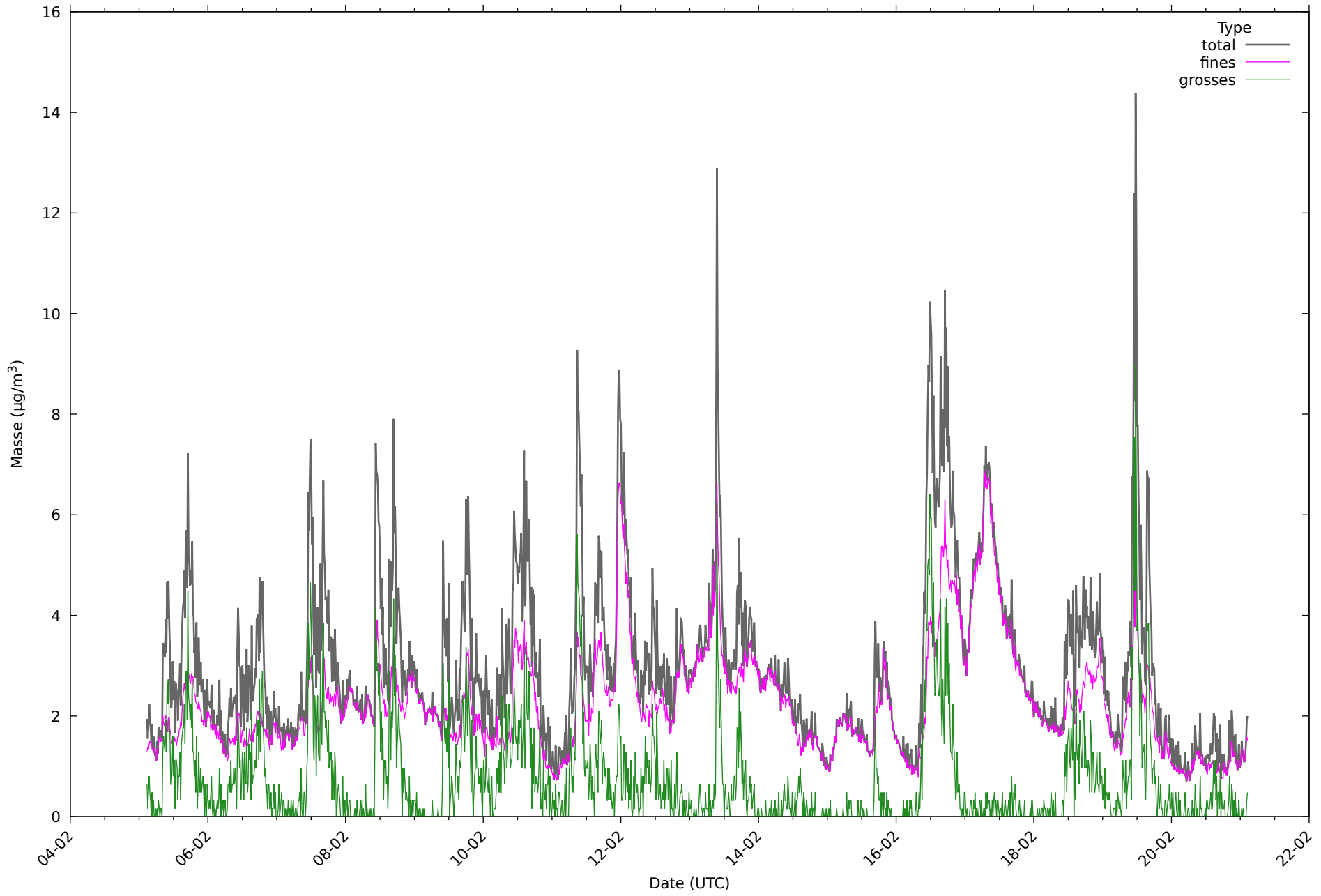
Particules sur 12 jours au 21/02/2026
