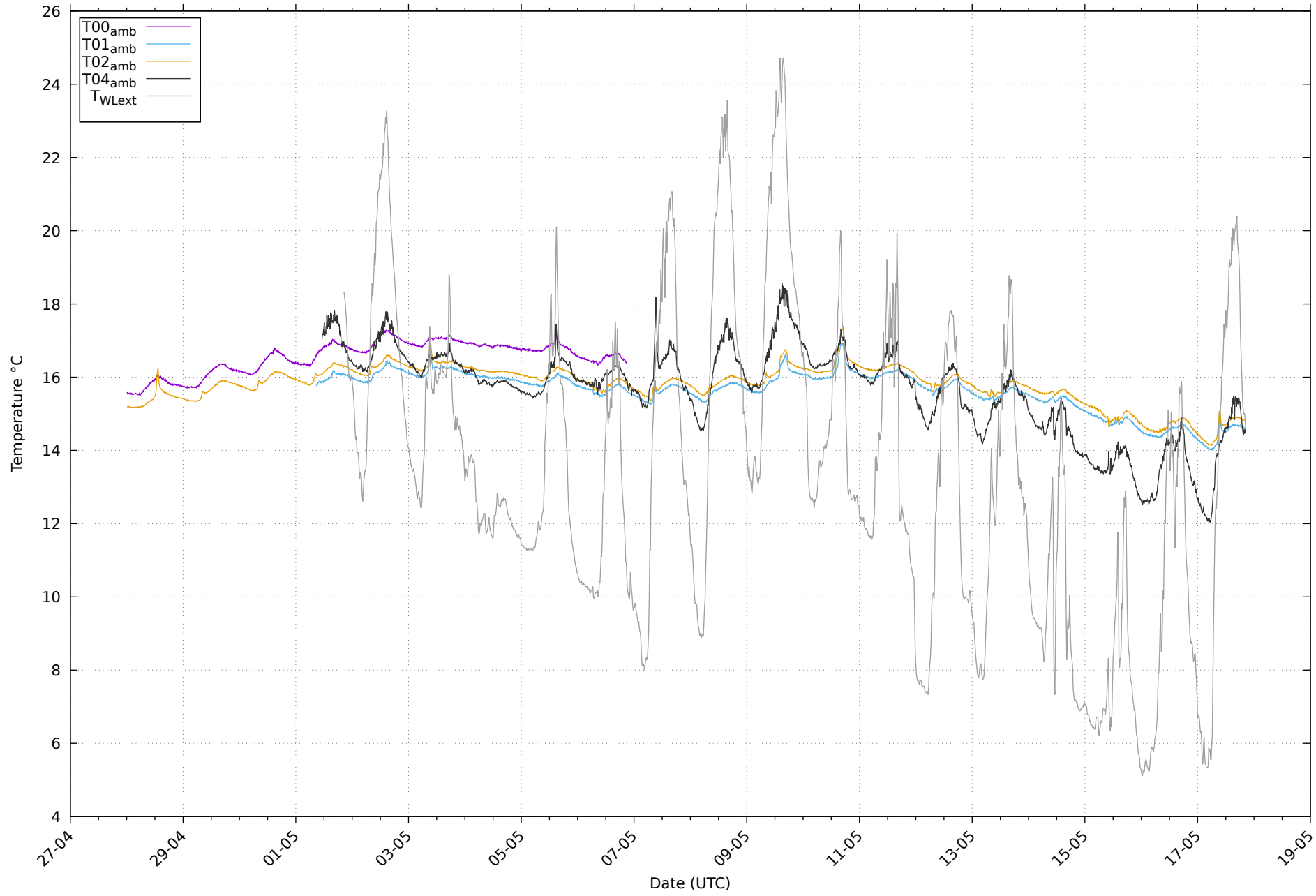
Températures au 17/05/2026
