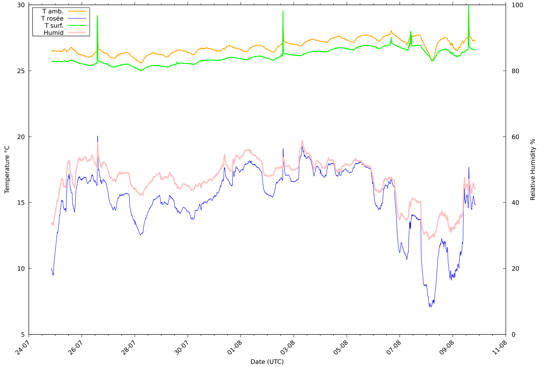
Températures et humidité sur 12 jours au 09/08/2026
