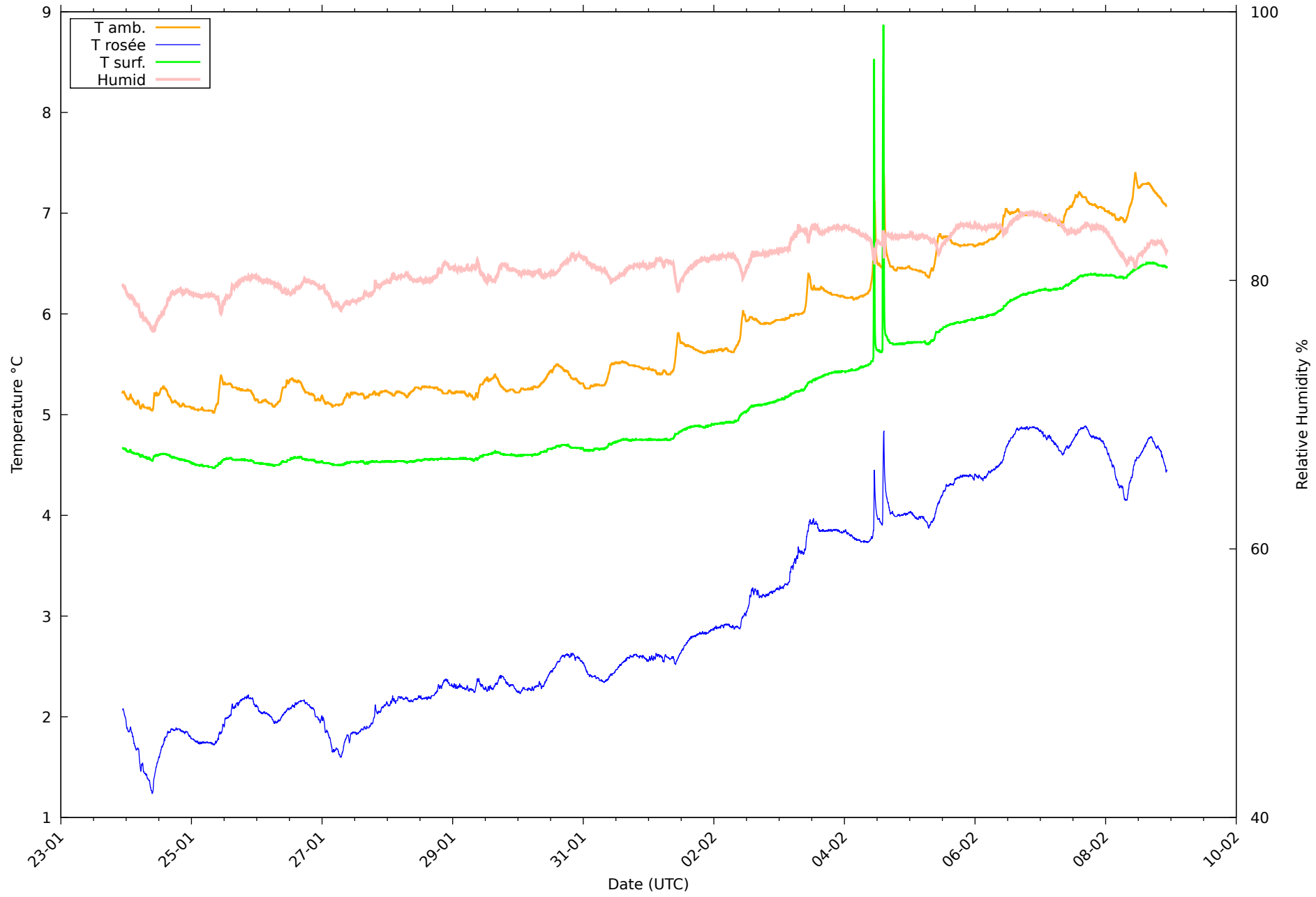
Températures et humidité sur 12 jours au 08/02/2026
