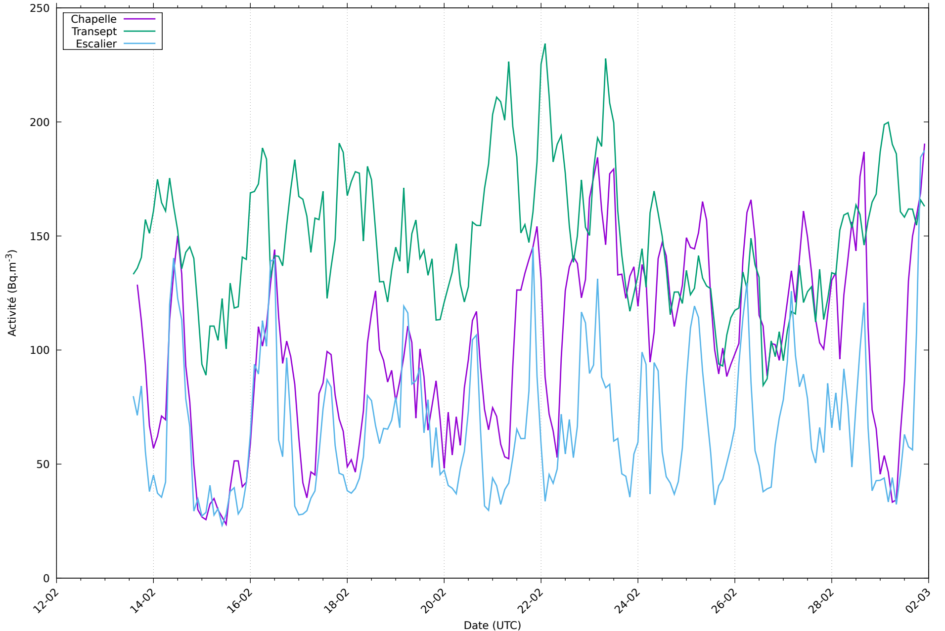
Radon sur 2 semaines au 01/03/2026
