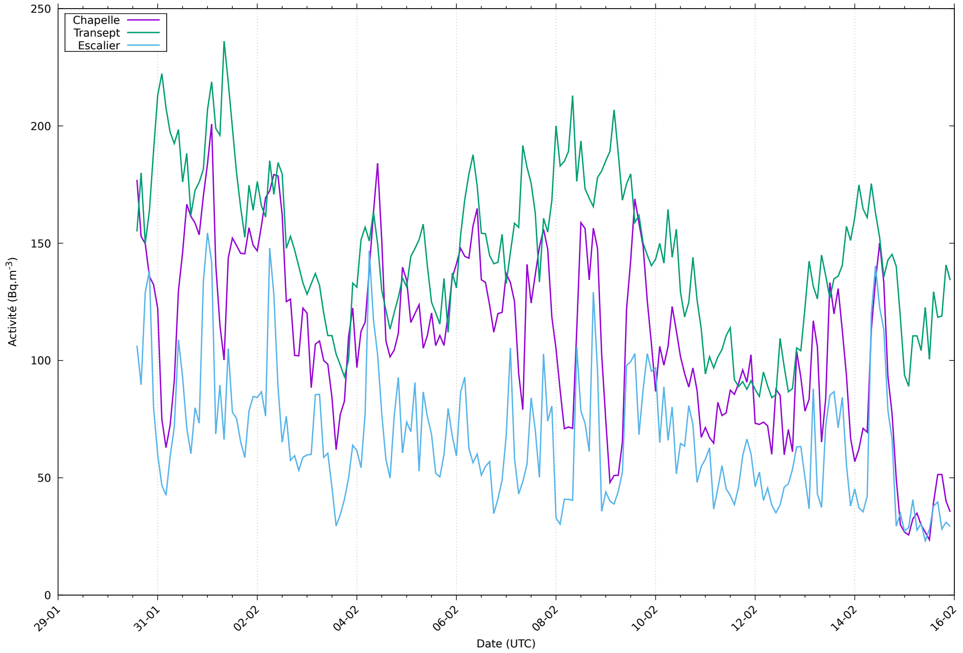
Radon sur 2 semaines au 15/02/2026
