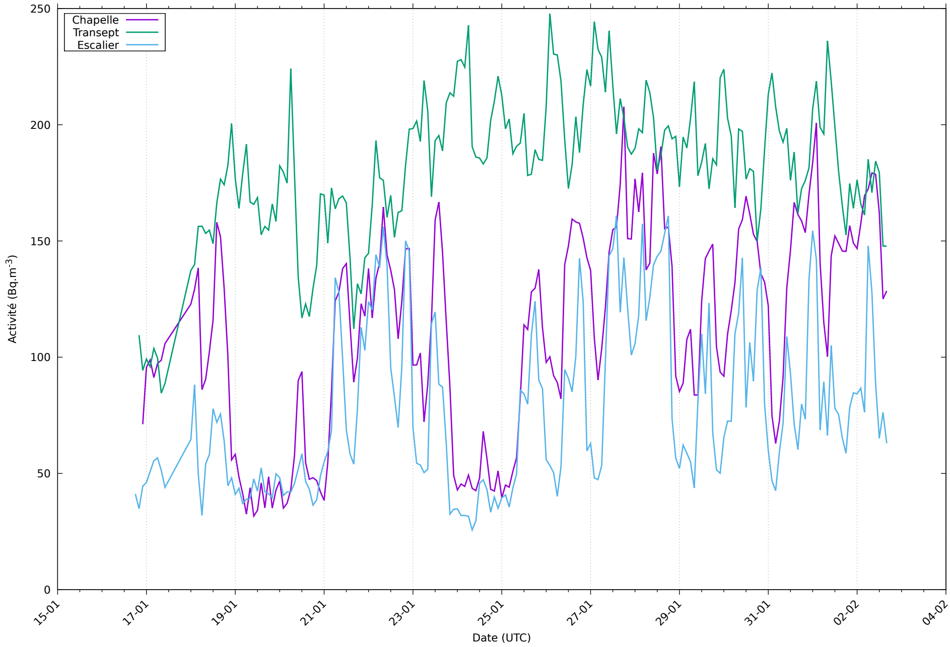
Radon sur 2 semaines au 02/02/2026
