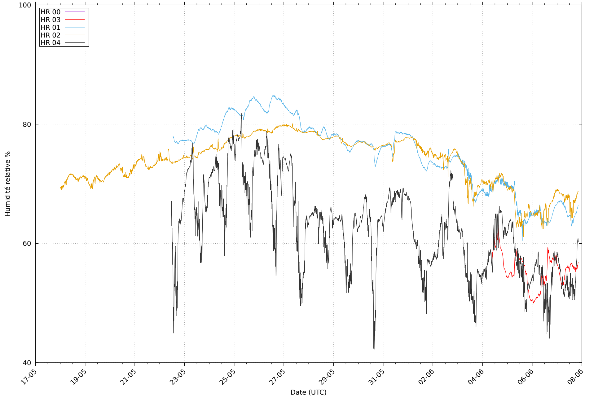
Humidités relatives au 07/06/2026
