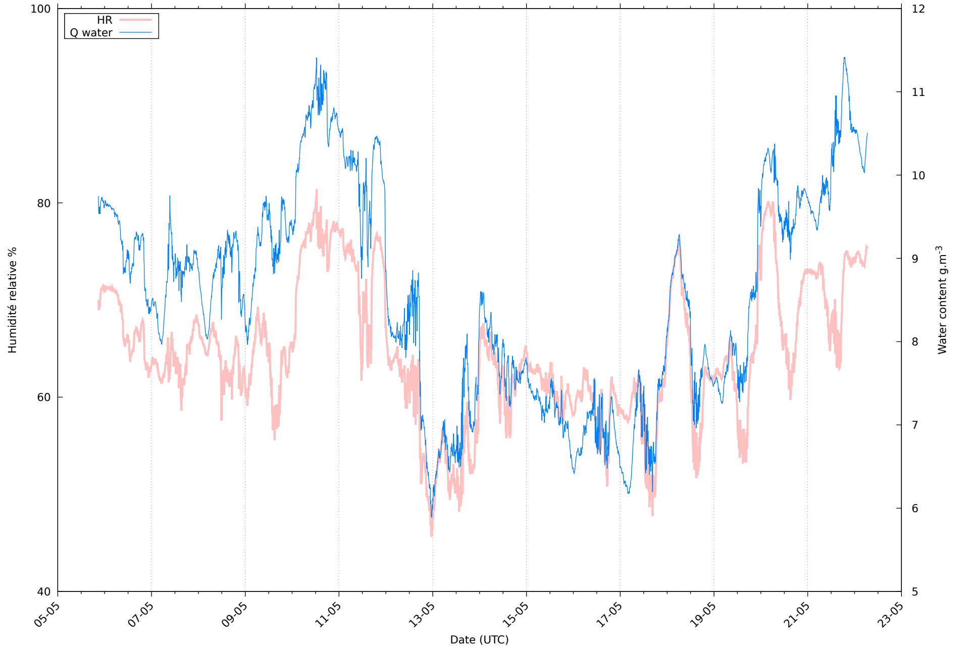
Humidité au 24/05/2026 pour RHT04
