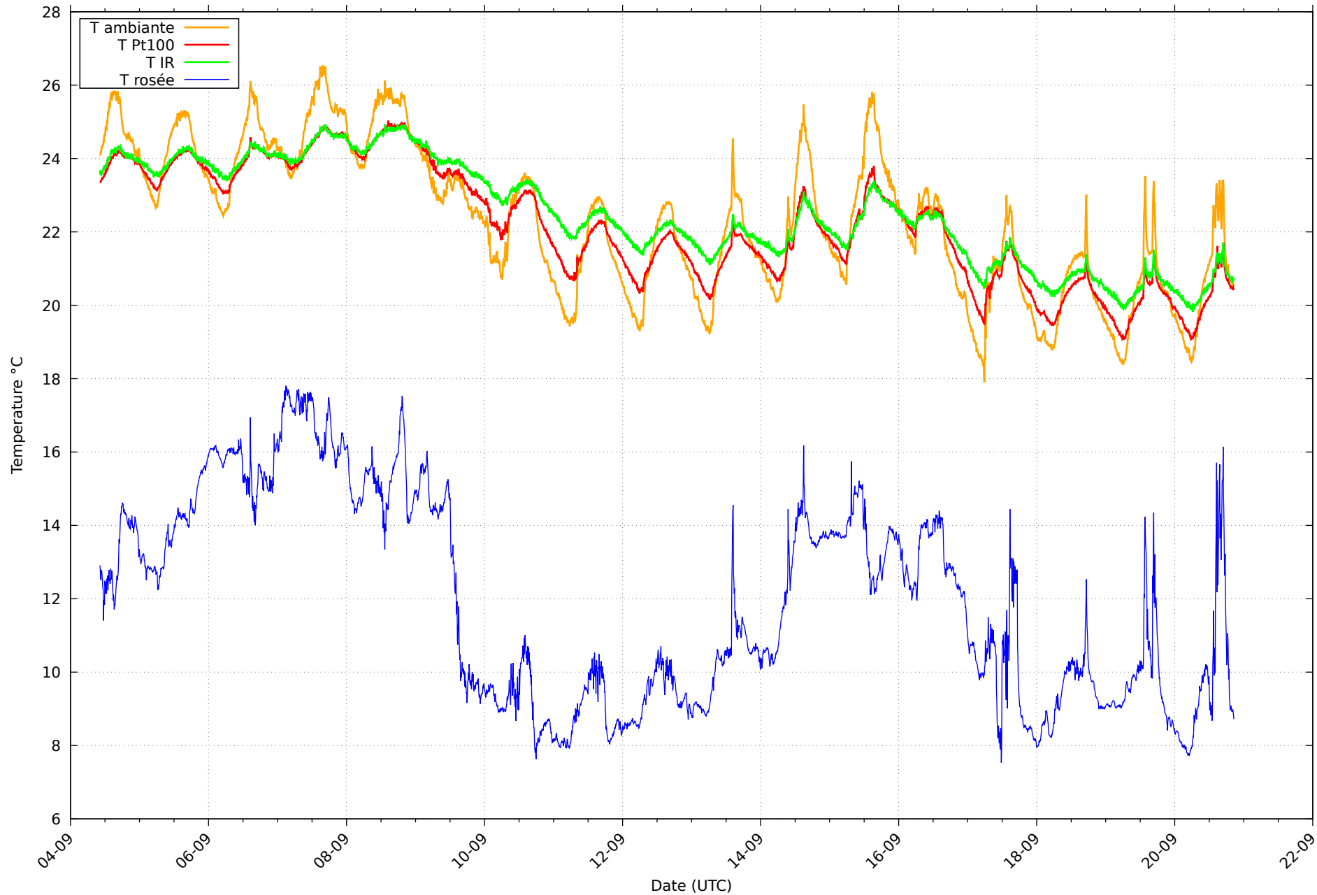
Température et rosée au 20/09/2026 pour RHT04
