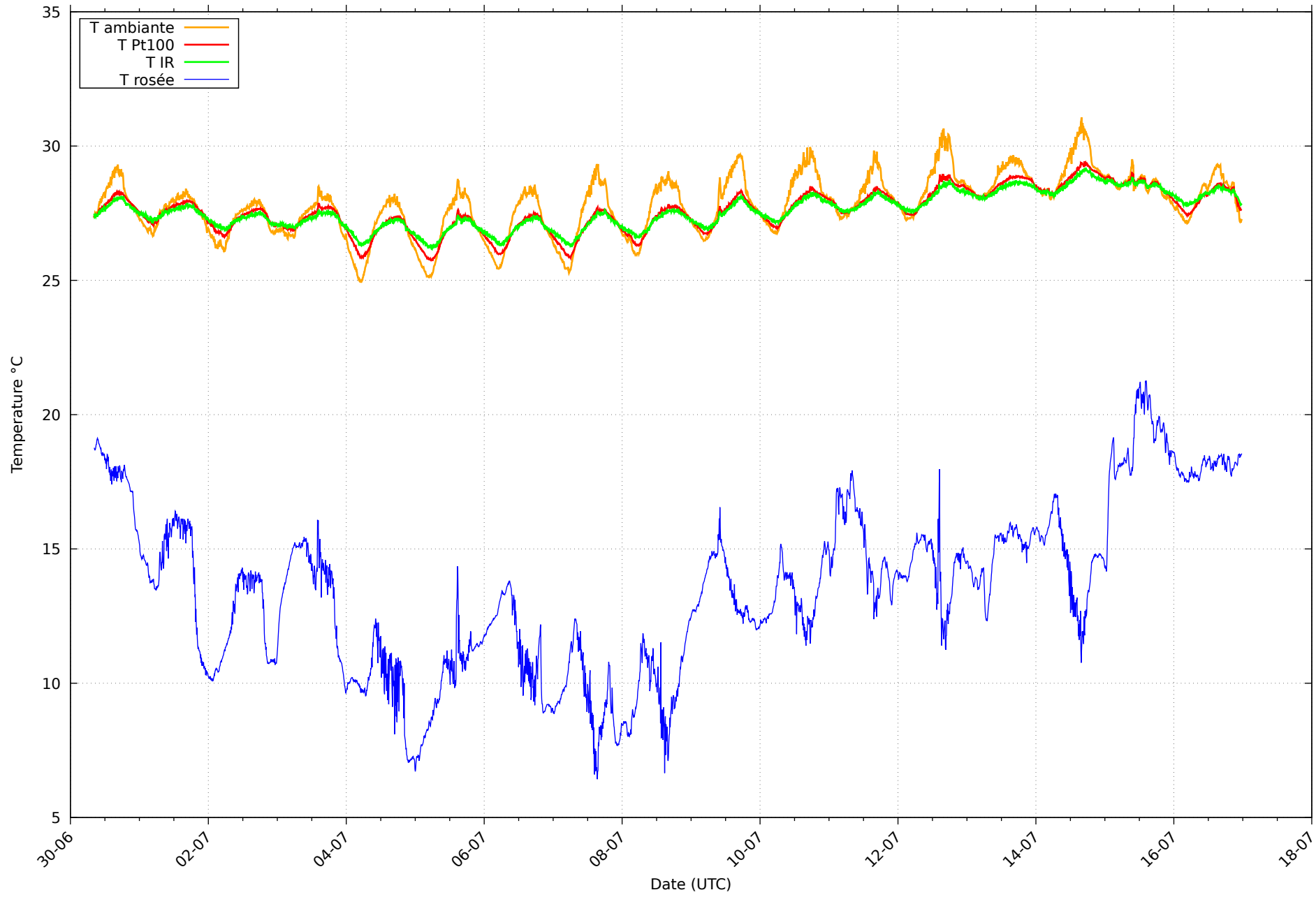
Température et rosée au 19/07/2026 pour RHT04
