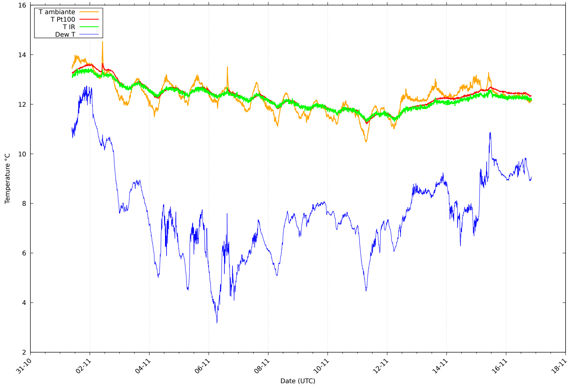
Température et rosée au 16/11/2025 pour RHT04
