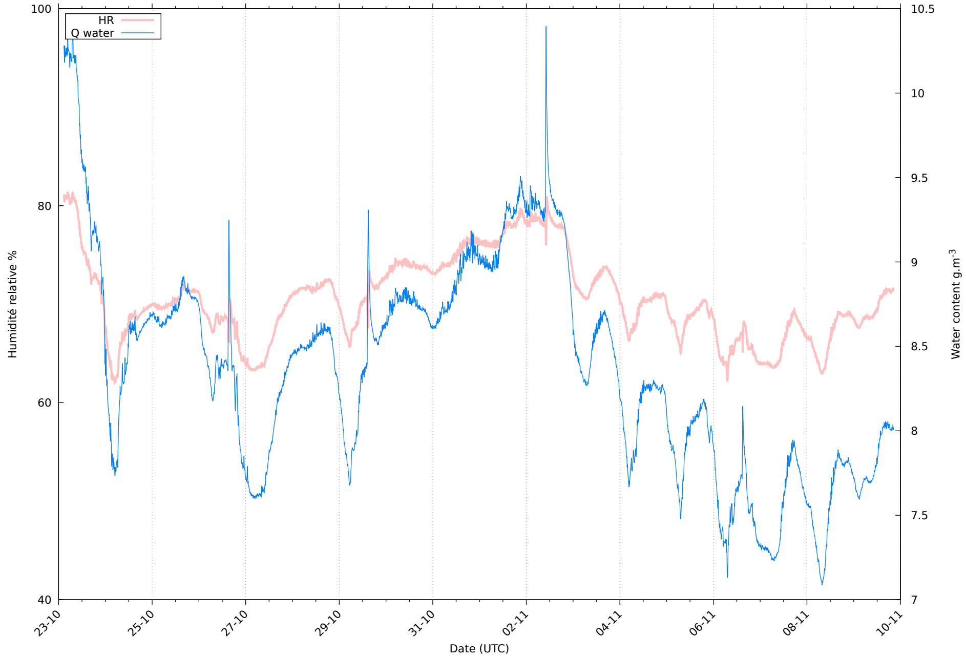
Humidité au 09/11/2025 pour RHT03
