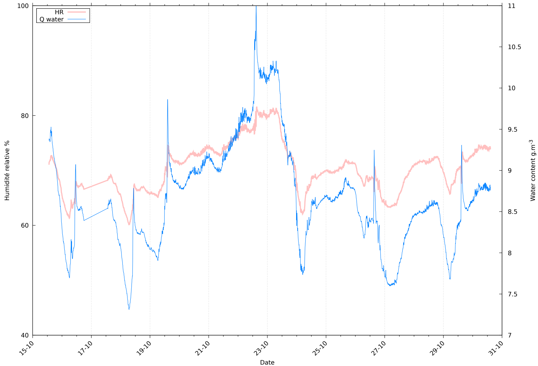
Humidité au 30/10/2025 pour RHT03
