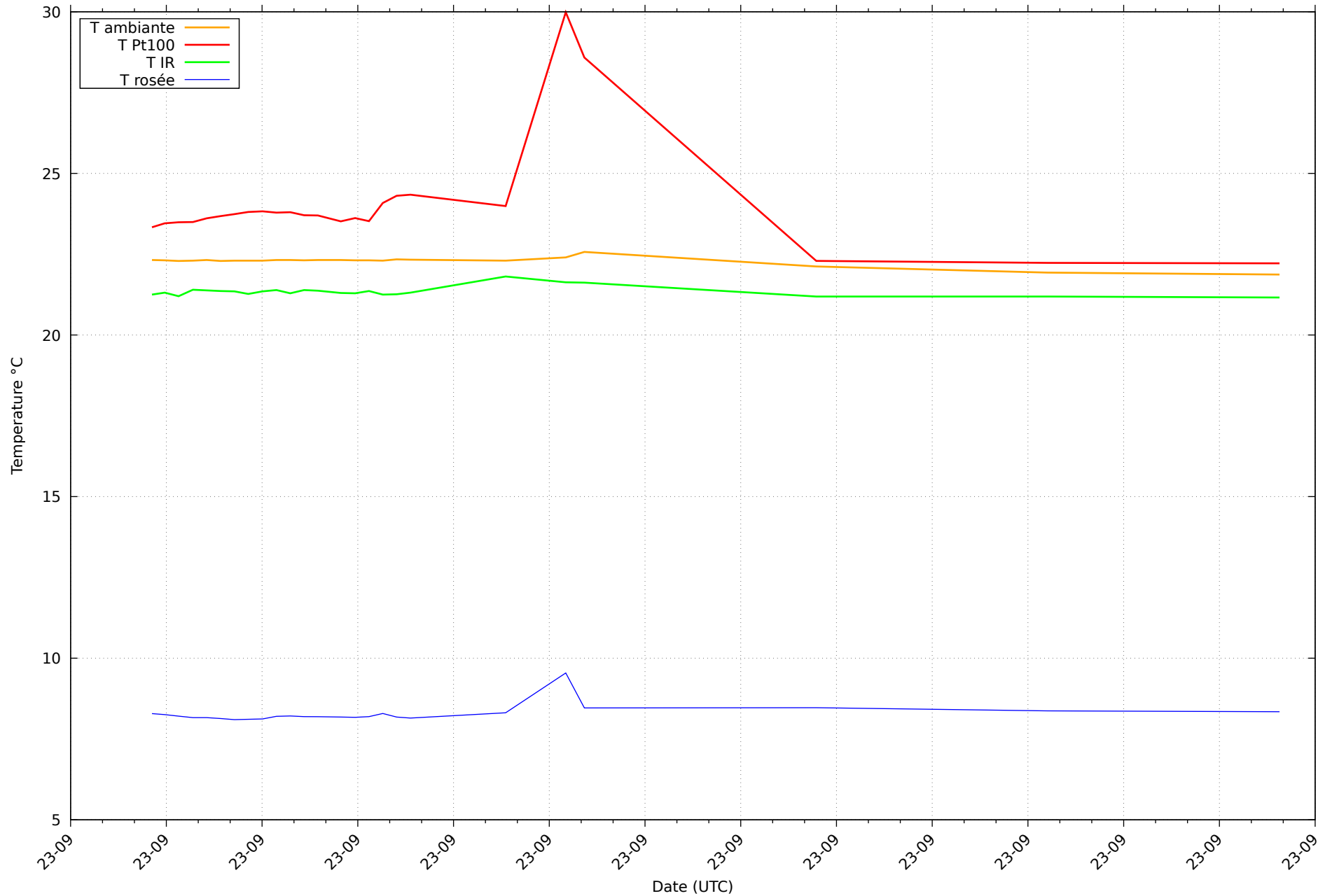
Température et rosée au 27/09/2026 pour RHT03
