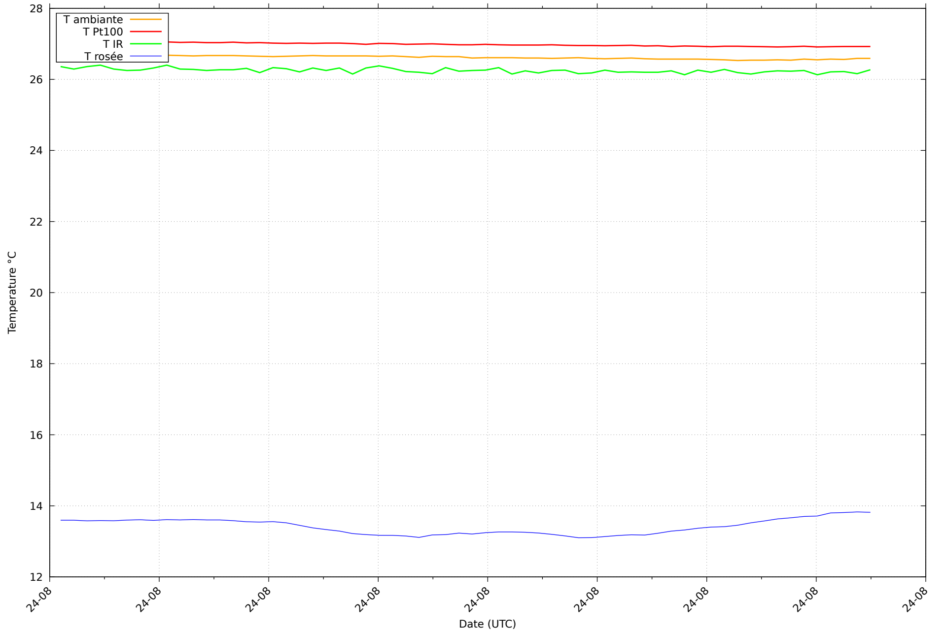
Température et rosée au 13/09/2026 pour RHT03
