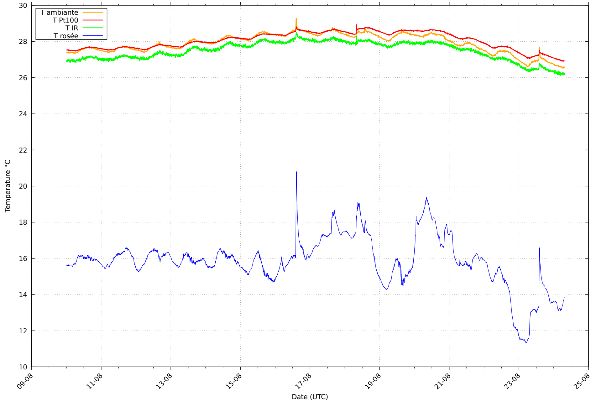
Température et rosée au 30/08/2026 pour RHT03
