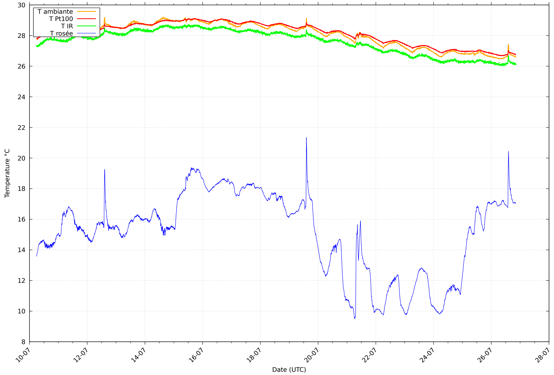
Température et rosée au 26/07/2026 pour RHT03
