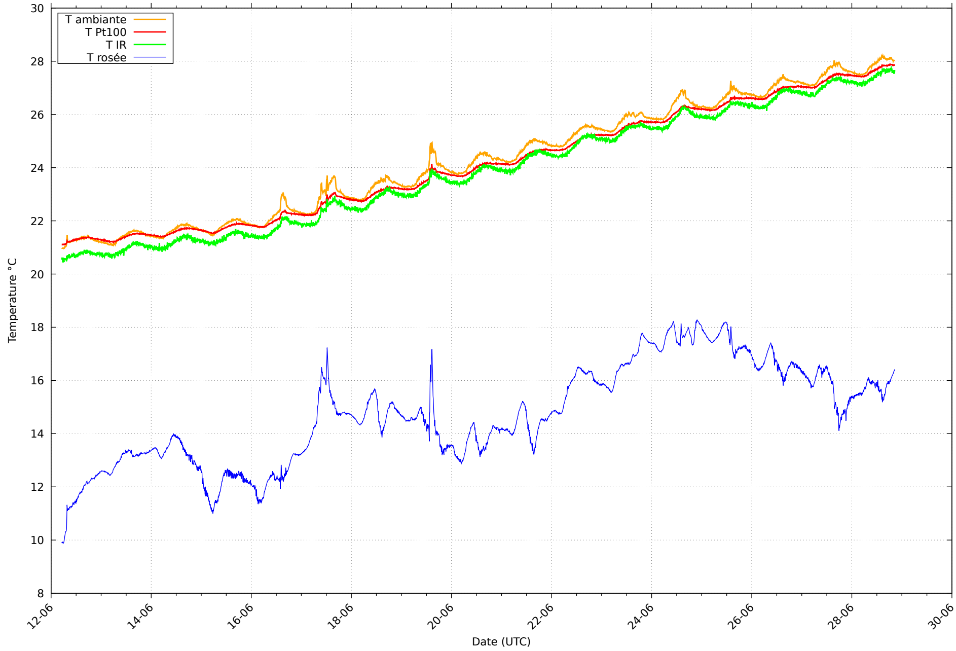
Température et rosée au 28/06/2026 pour RHT03
