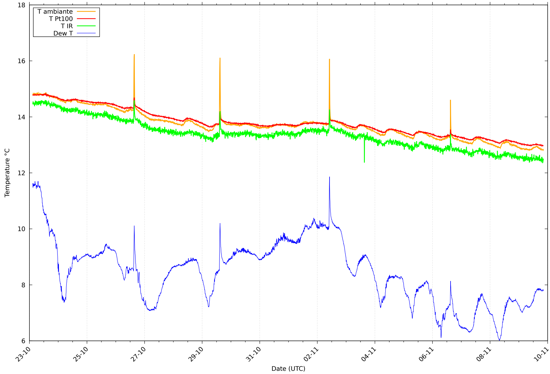
Température et rosée au 09/11/2025 pour RHT03
