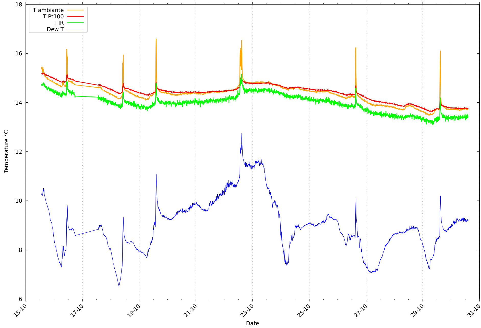
Température et rosée au 30/10/2025 pour RHT03
