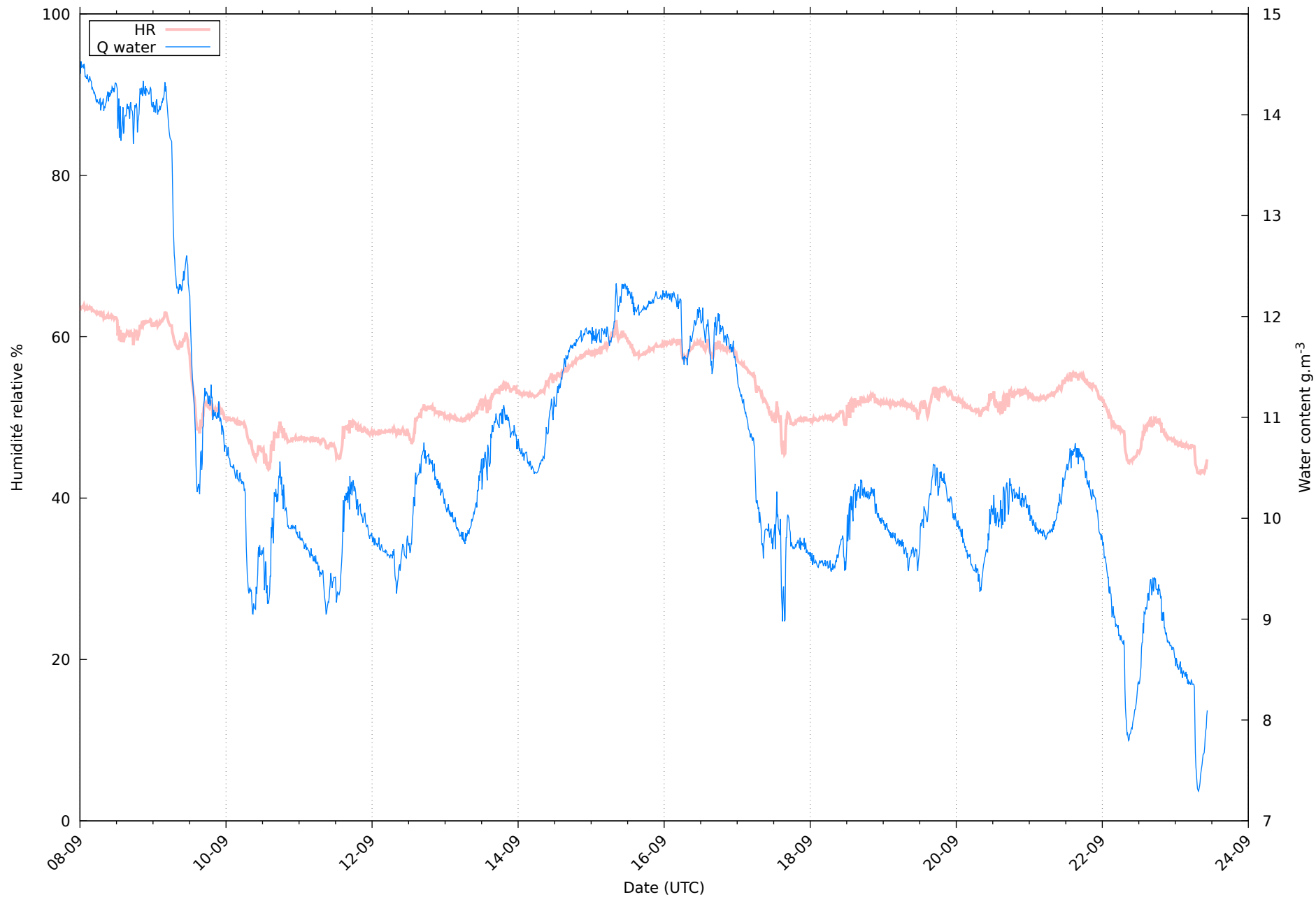
Humidité au 27/09/2026 pour RHT02
