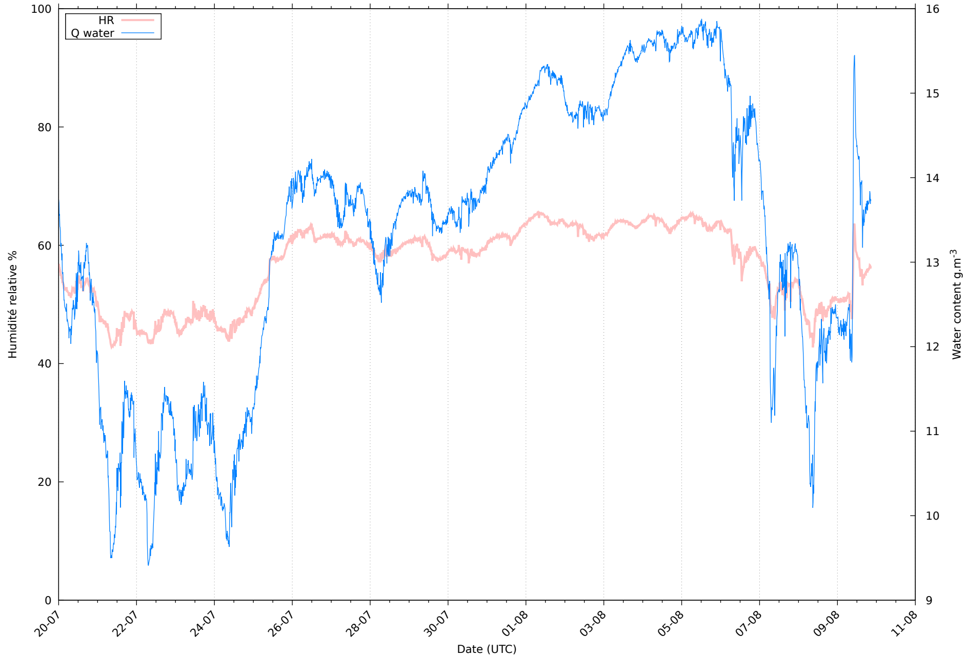
Humidité au 09/08/2026 pour RHT02
