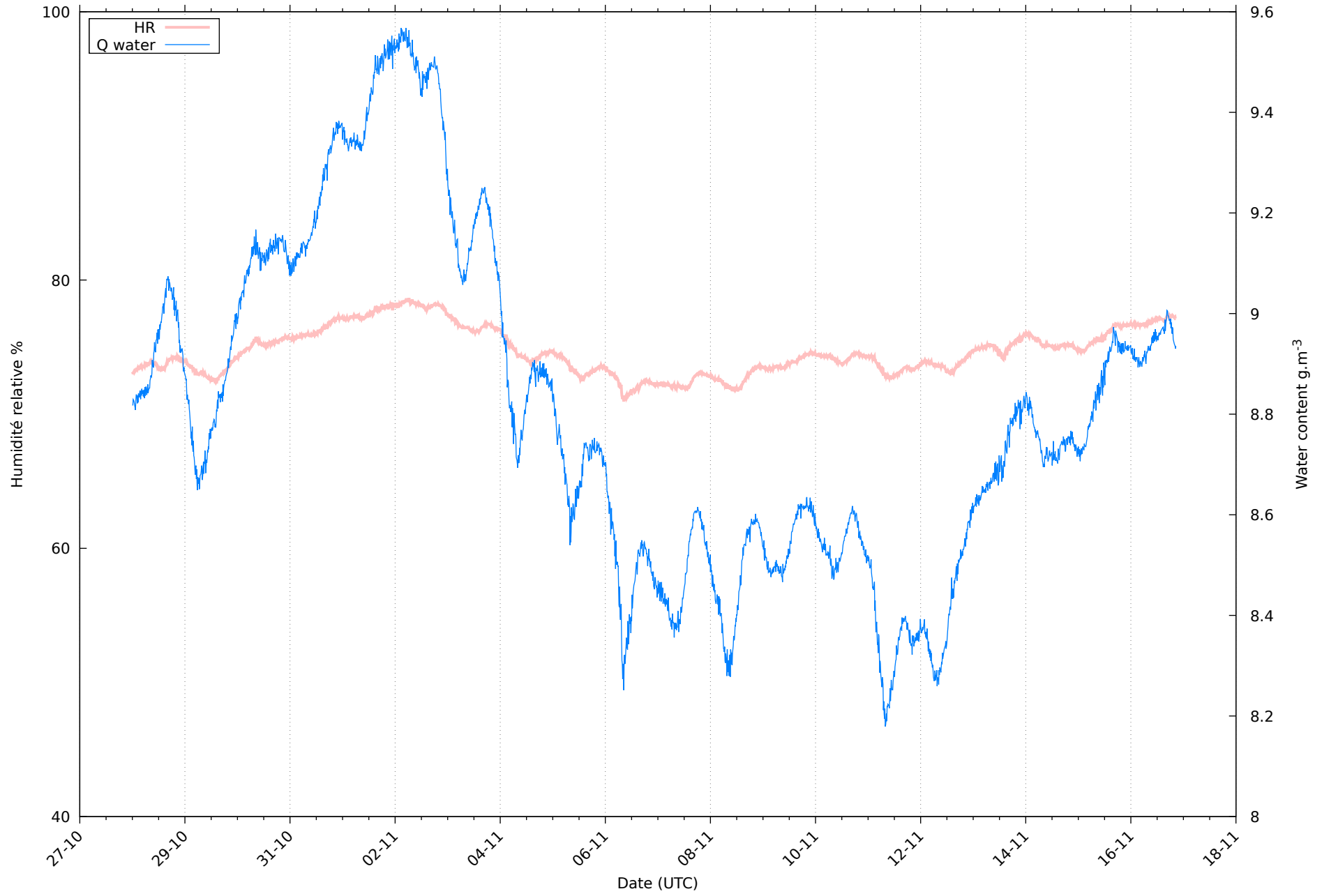
Humidité au 16/11/2025 pour RHT02
