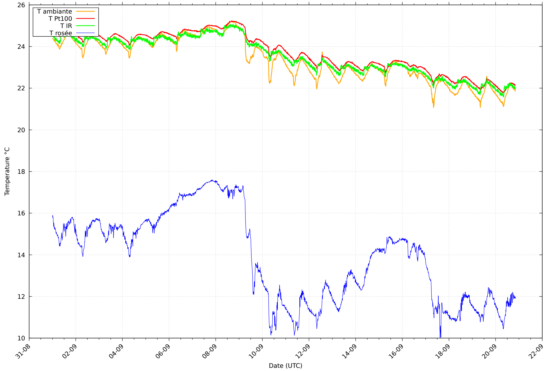
Température et rosée au 20/09/2026 pour RHT02
