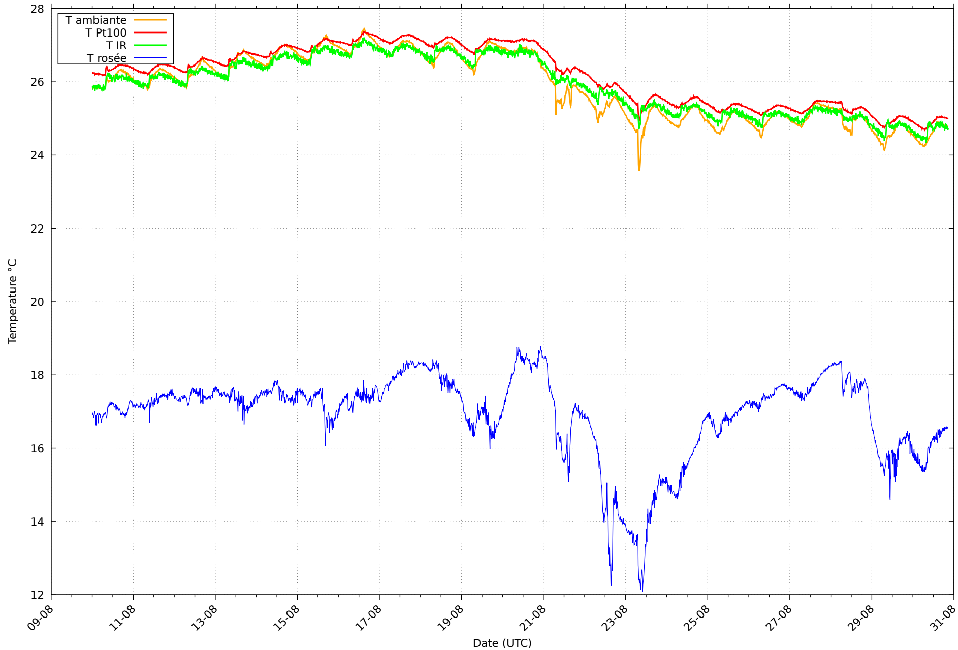
Température et rosée au 30/08/2026 pour RHT02
