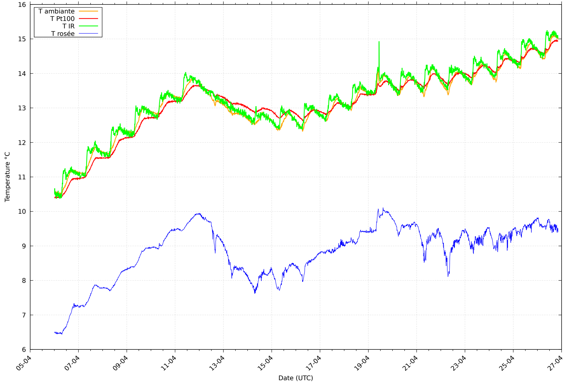
Température et rosée au 26/04/2026 pour RHT02
