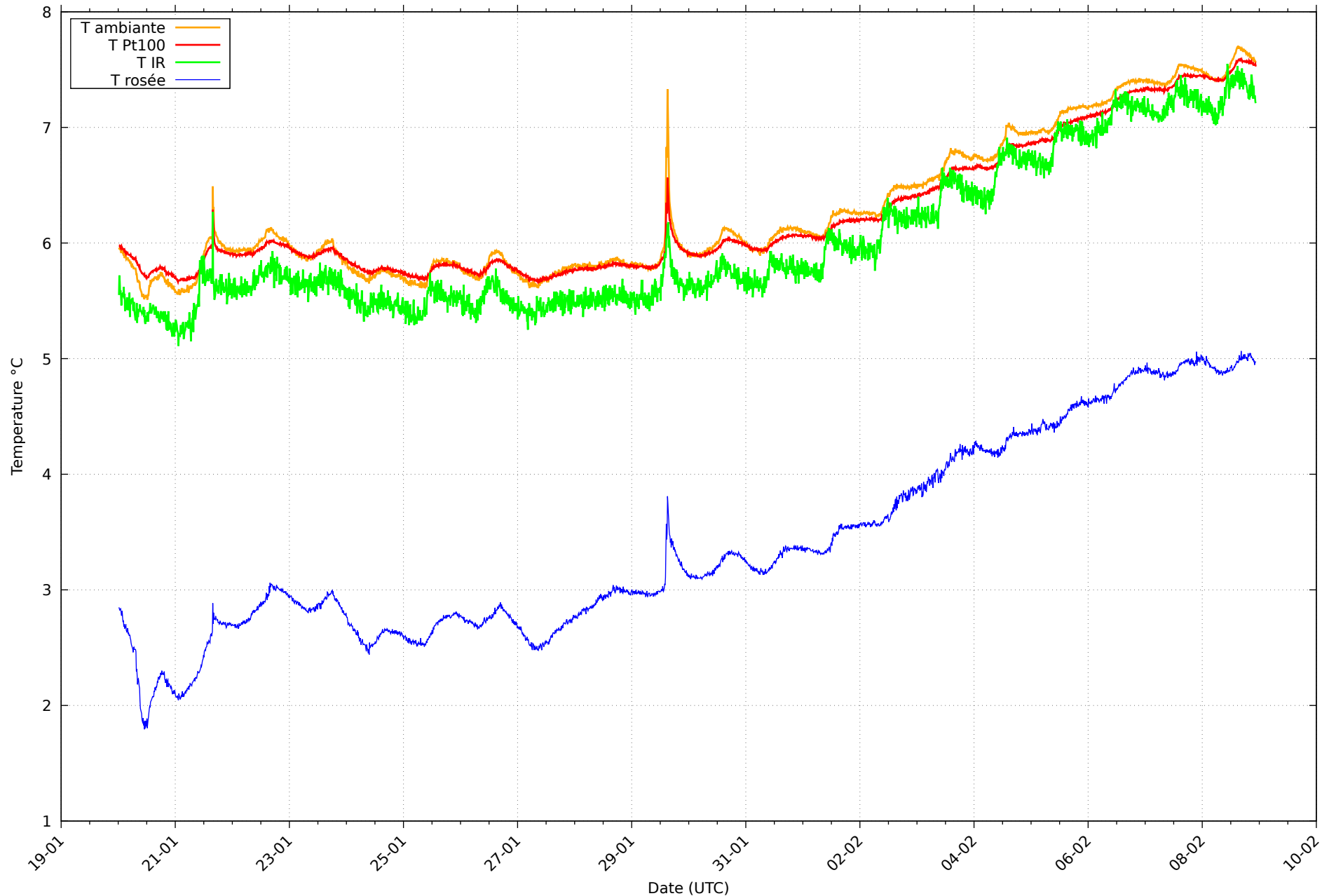
Température et rosée au 08/02/2026 pour RHT02
