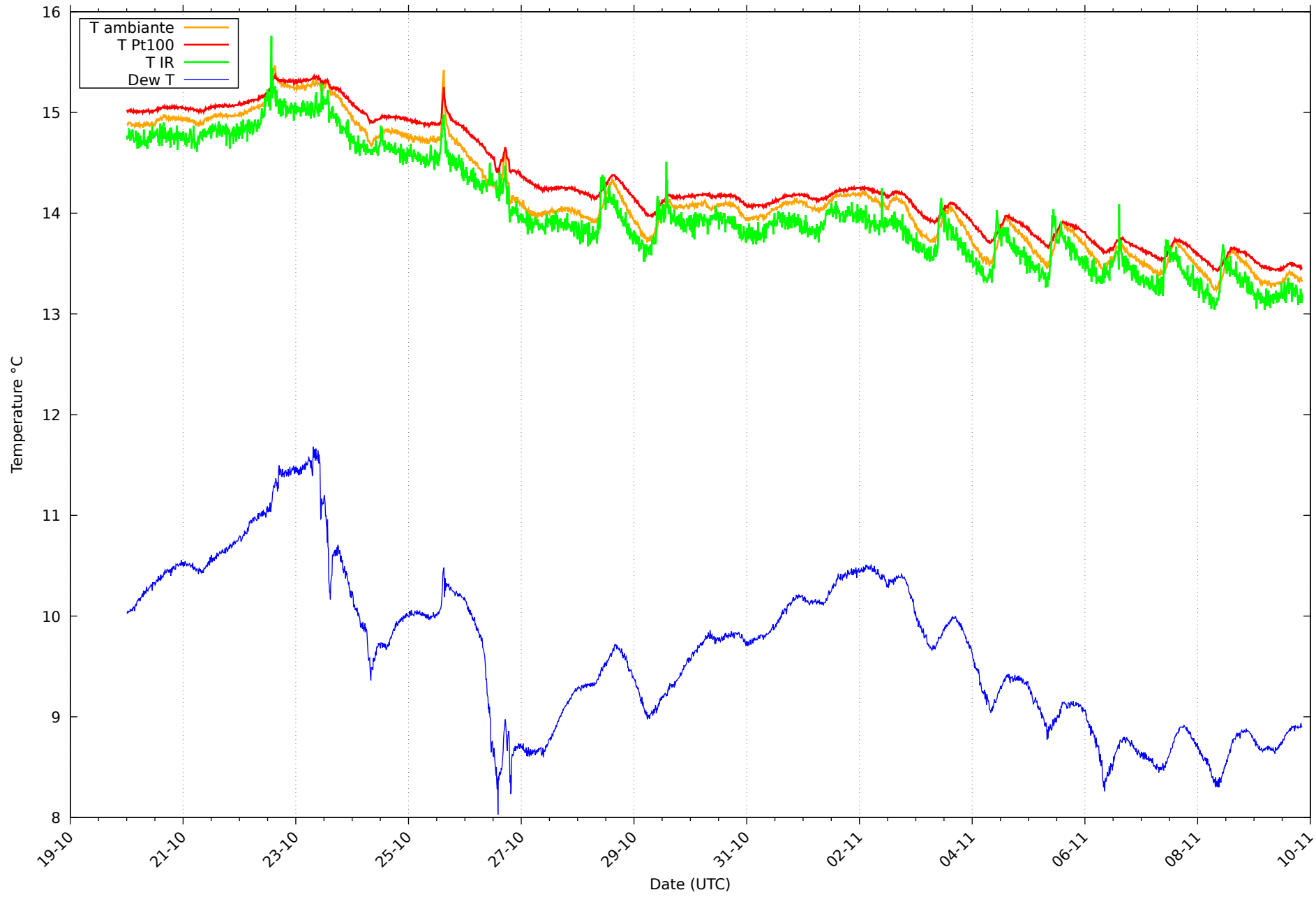
Température et rosée au 09/11/2025 pour RHT02
