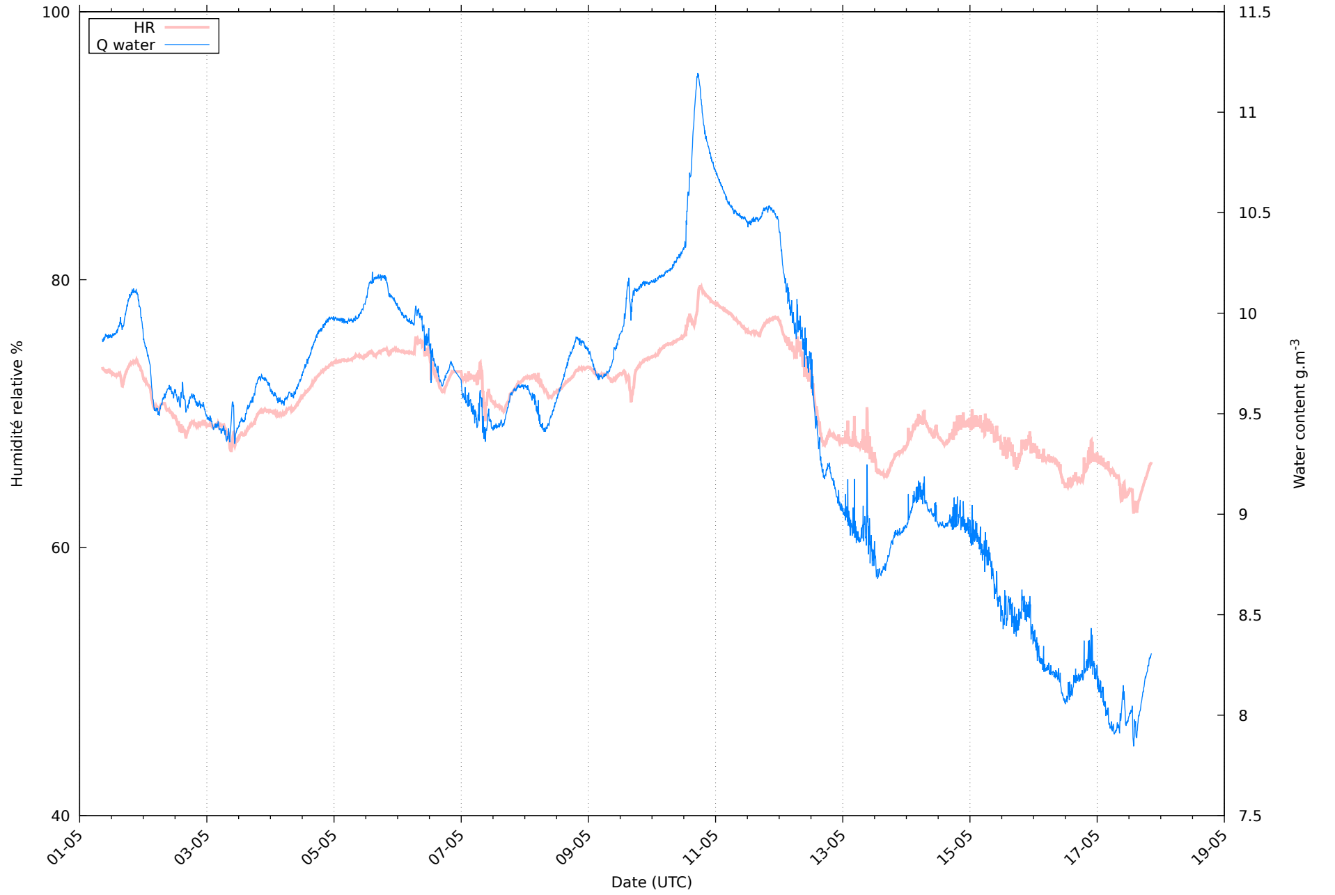
Humidité au 17/05/2026 pour RHT01
