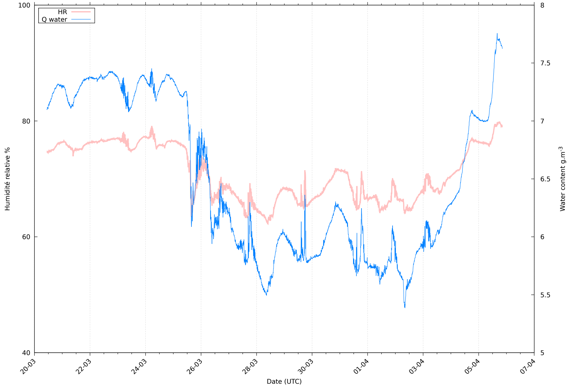
Humidité au 05/04/2026 pour RHT01
