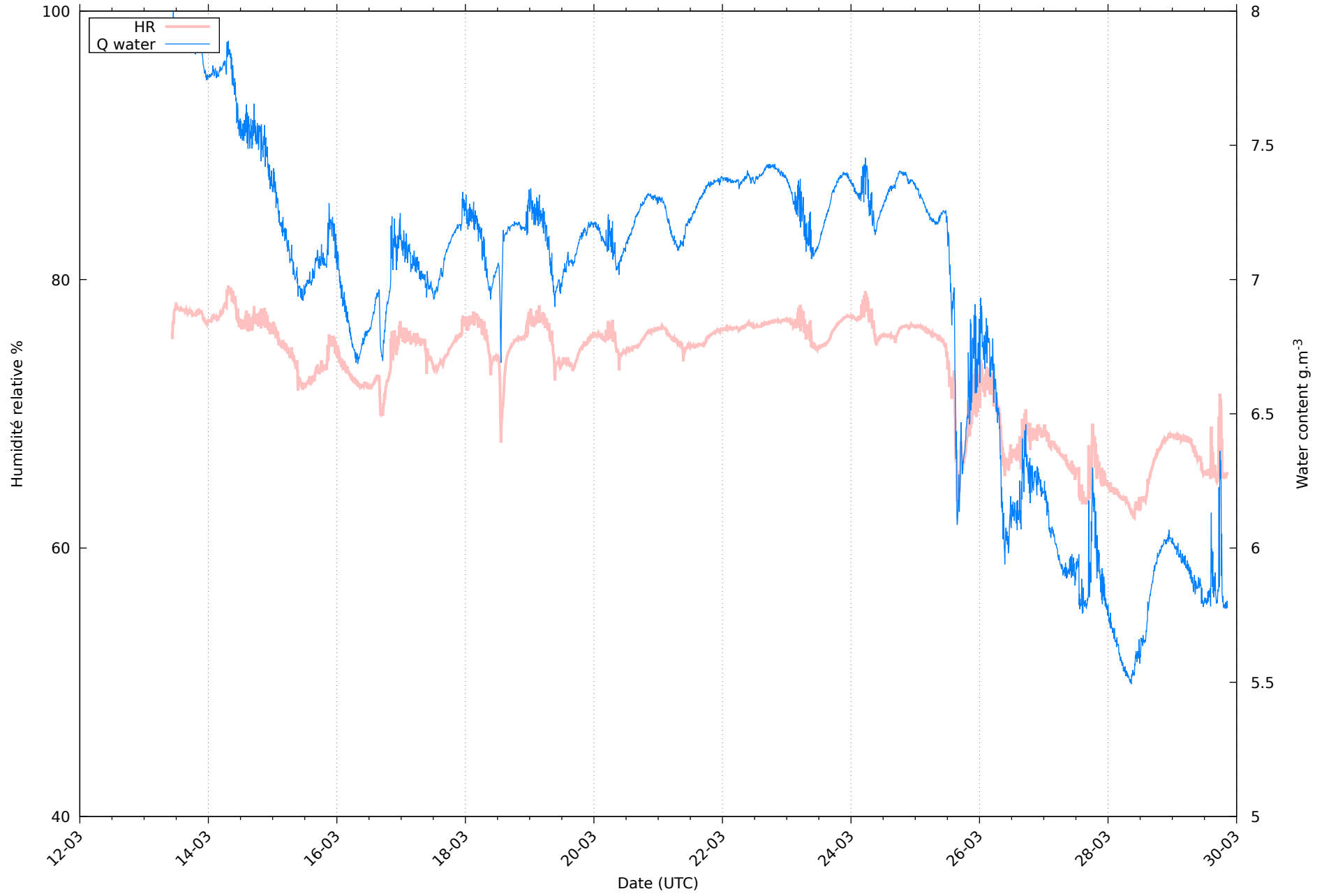
Humidité au 29/03/2026 pour RHT01
