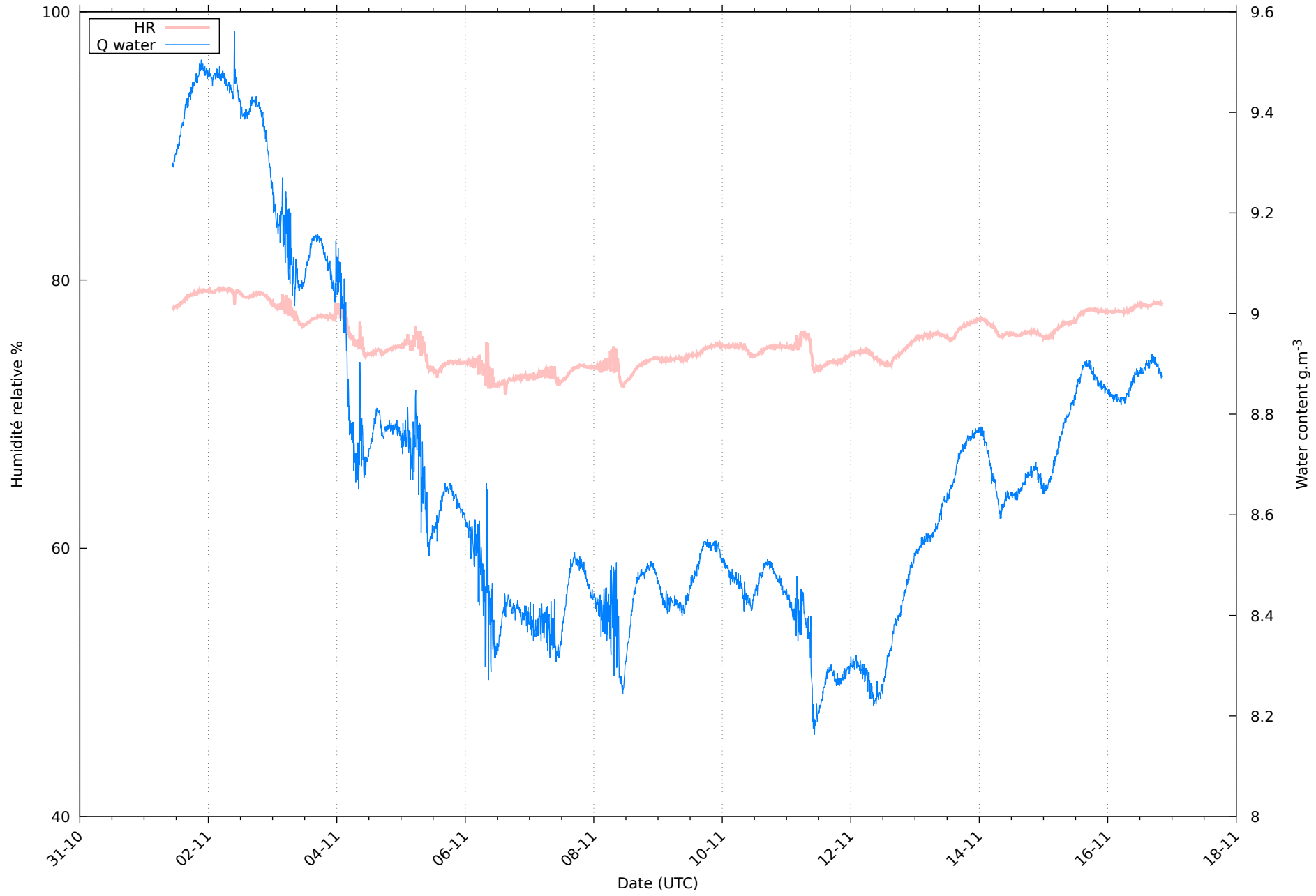
Humidité au 16/11/2025 pour RHT01
