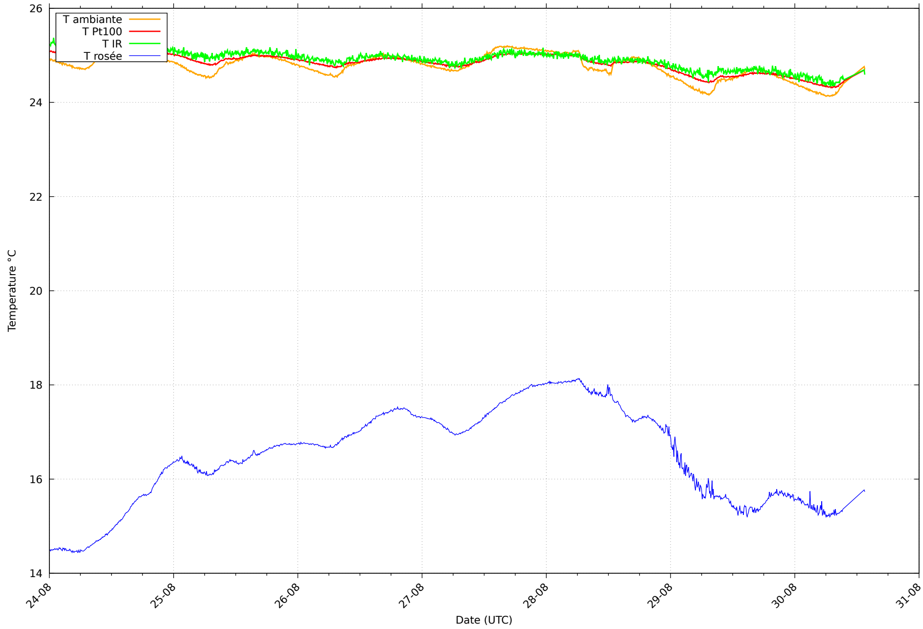
Température et rosée au 13/09/2026 pour RHT01
