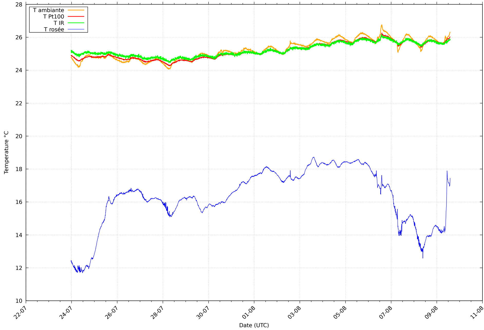
Température et rosée au 09/08/2026 pour RHT01
