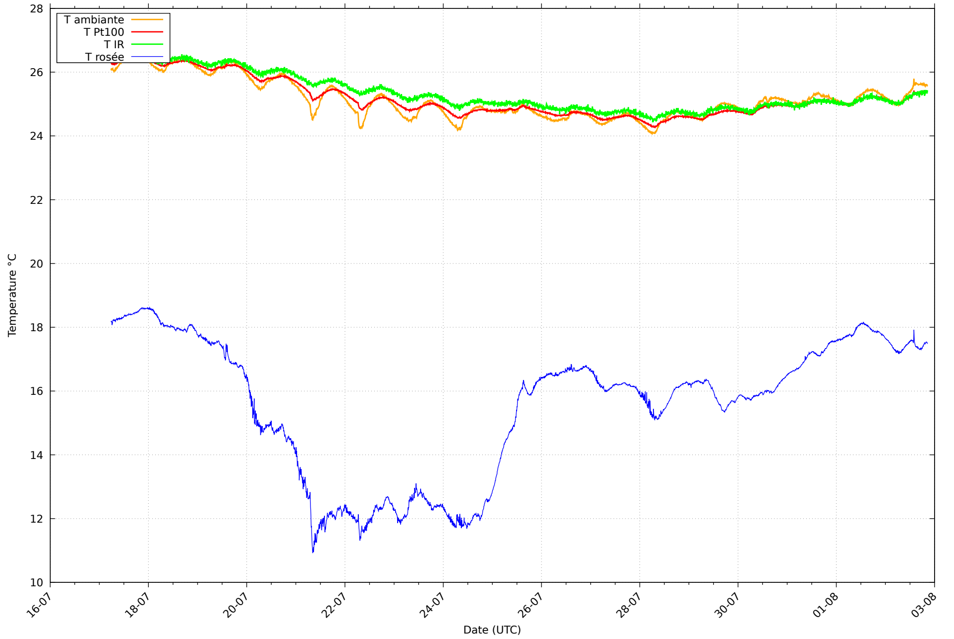
Température et rosée au 02/08/2026 pour RHT01
