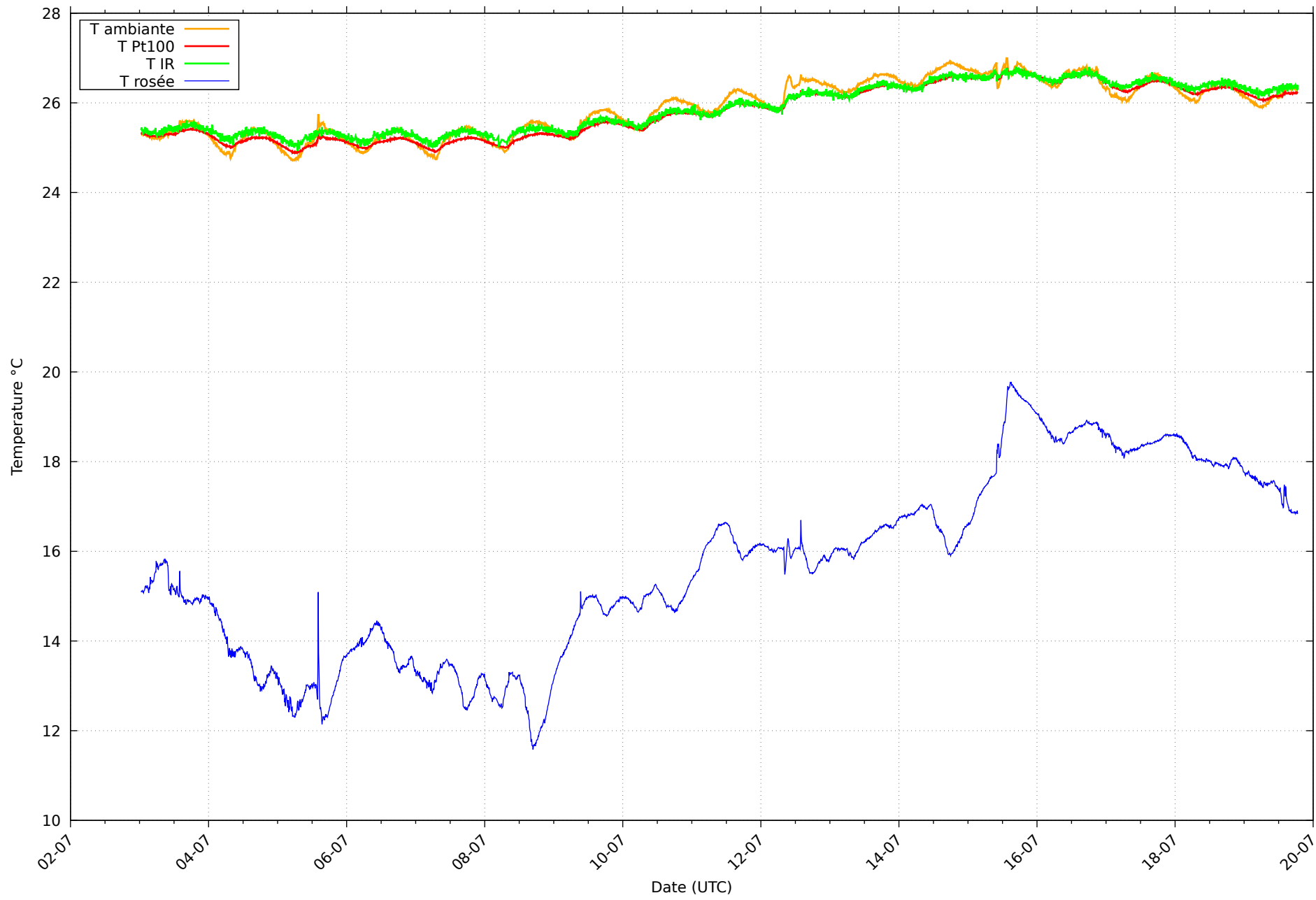
Température et rosée au 19/07/2026 pour RHT01
