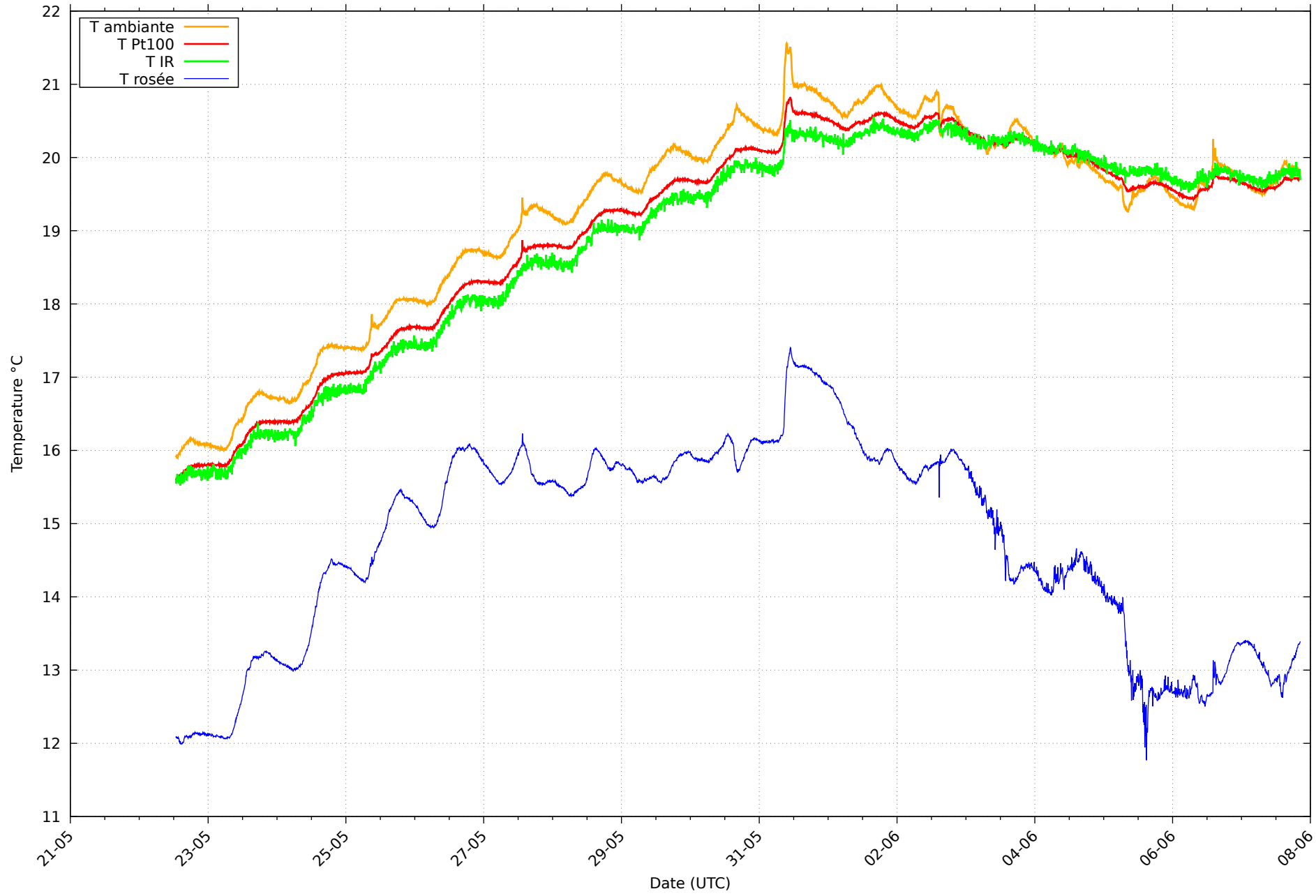
Température et rosée au 07/06/2026 pour RHT01
