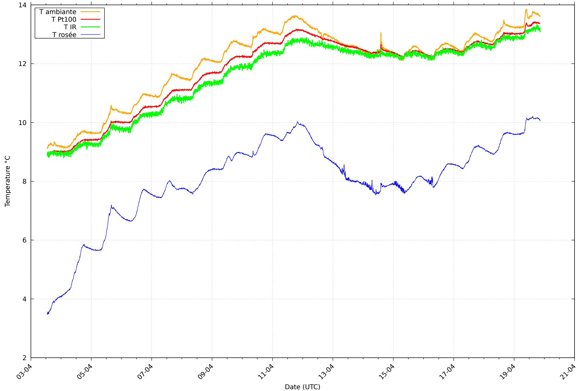
Température et rosée au 19/04/2026 pour RHT01
