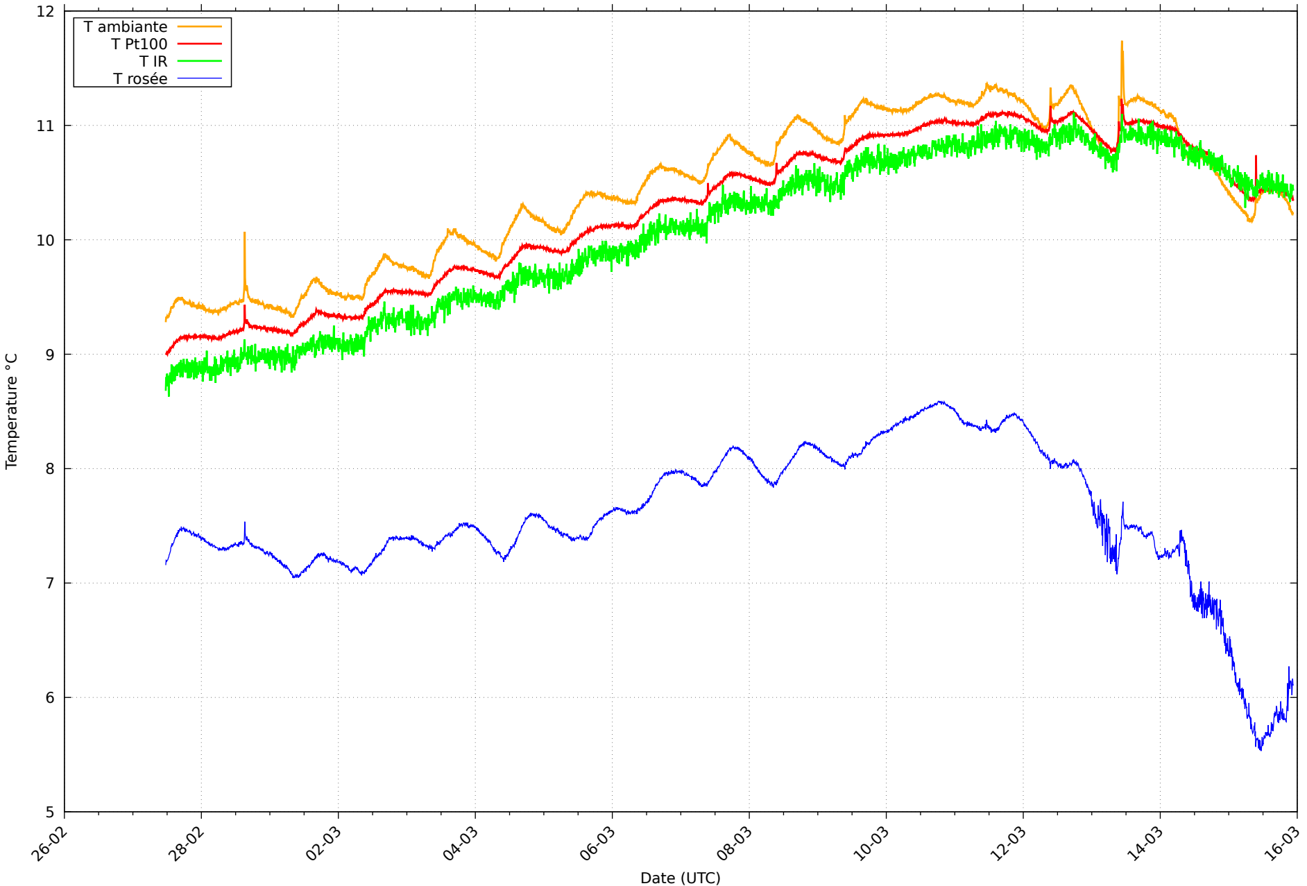
Température et rosée au 15/03/2026 pour RHT01
