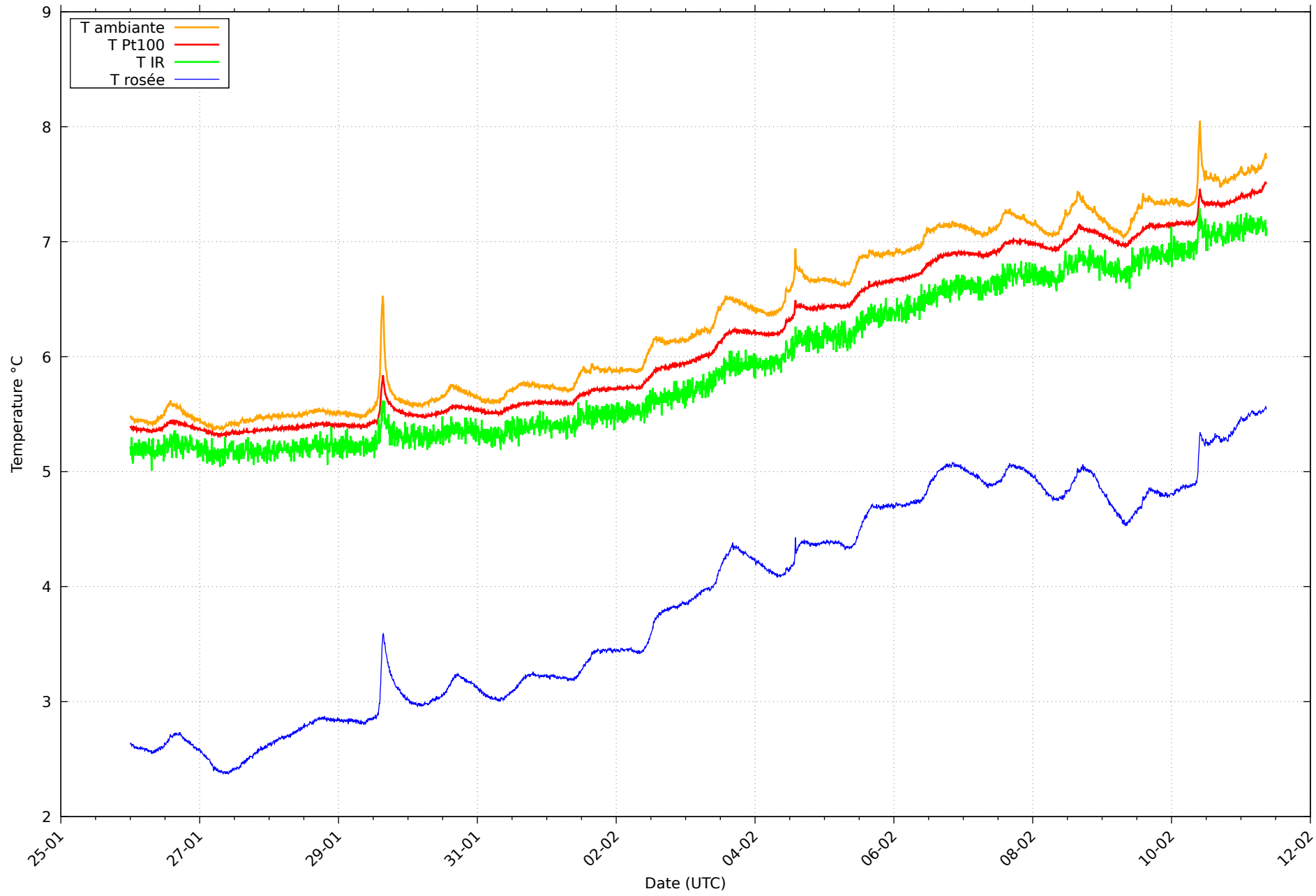
Température et rosée au 15/02/2026 pour RHT01
