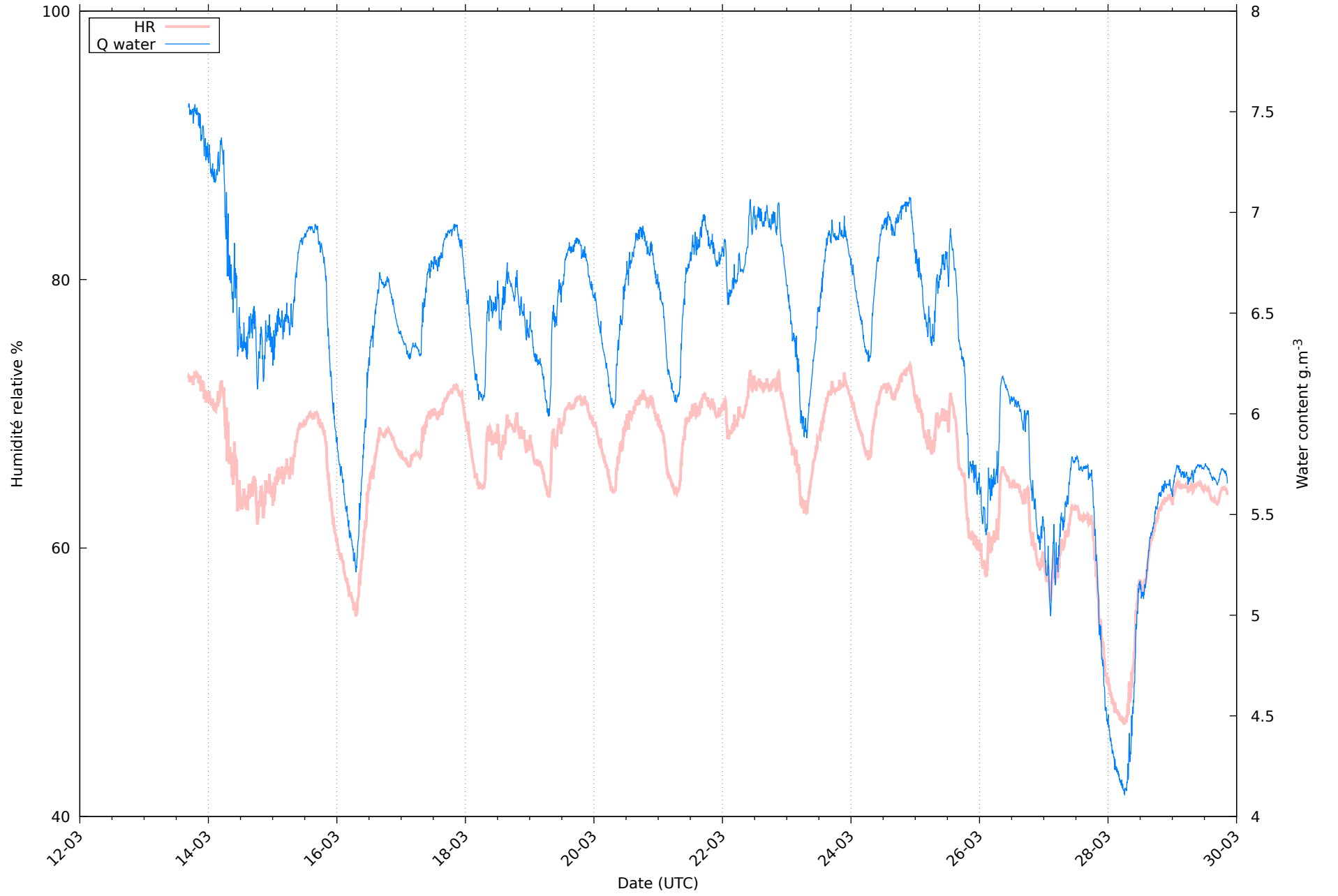
Humidité au 29/03/2026 pour RHT00
