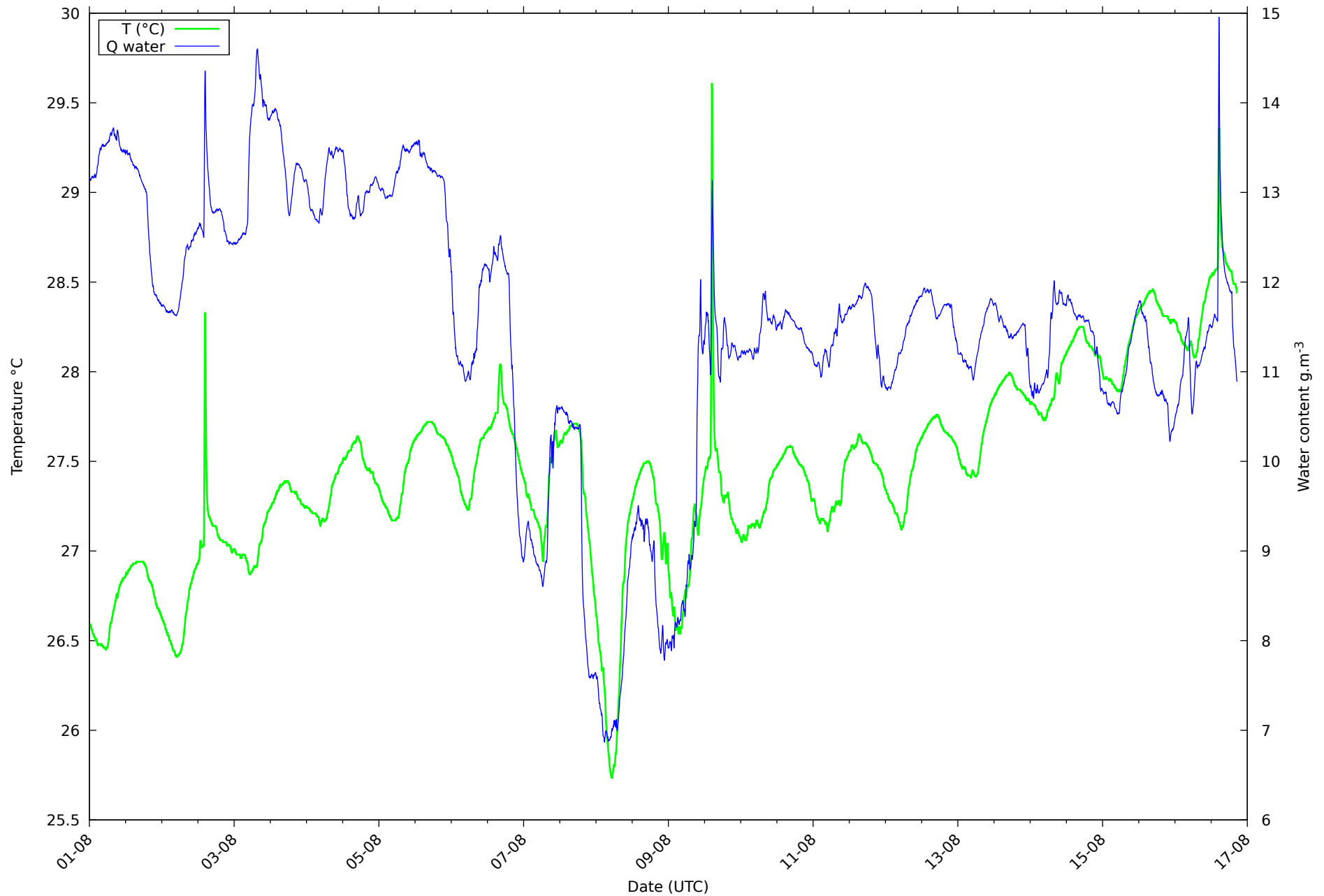
Températures et humidité sur 12 jours au 16/08/2026
