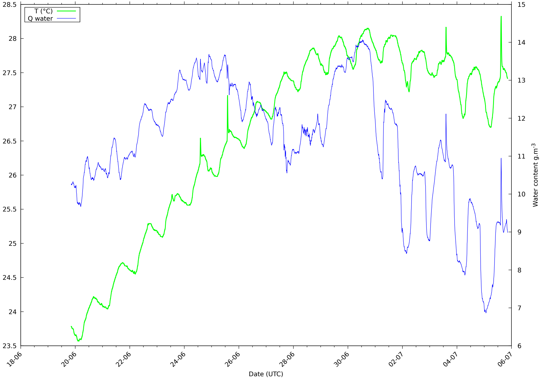
Températures et humidité sur 12 jours au 05/07/2026
