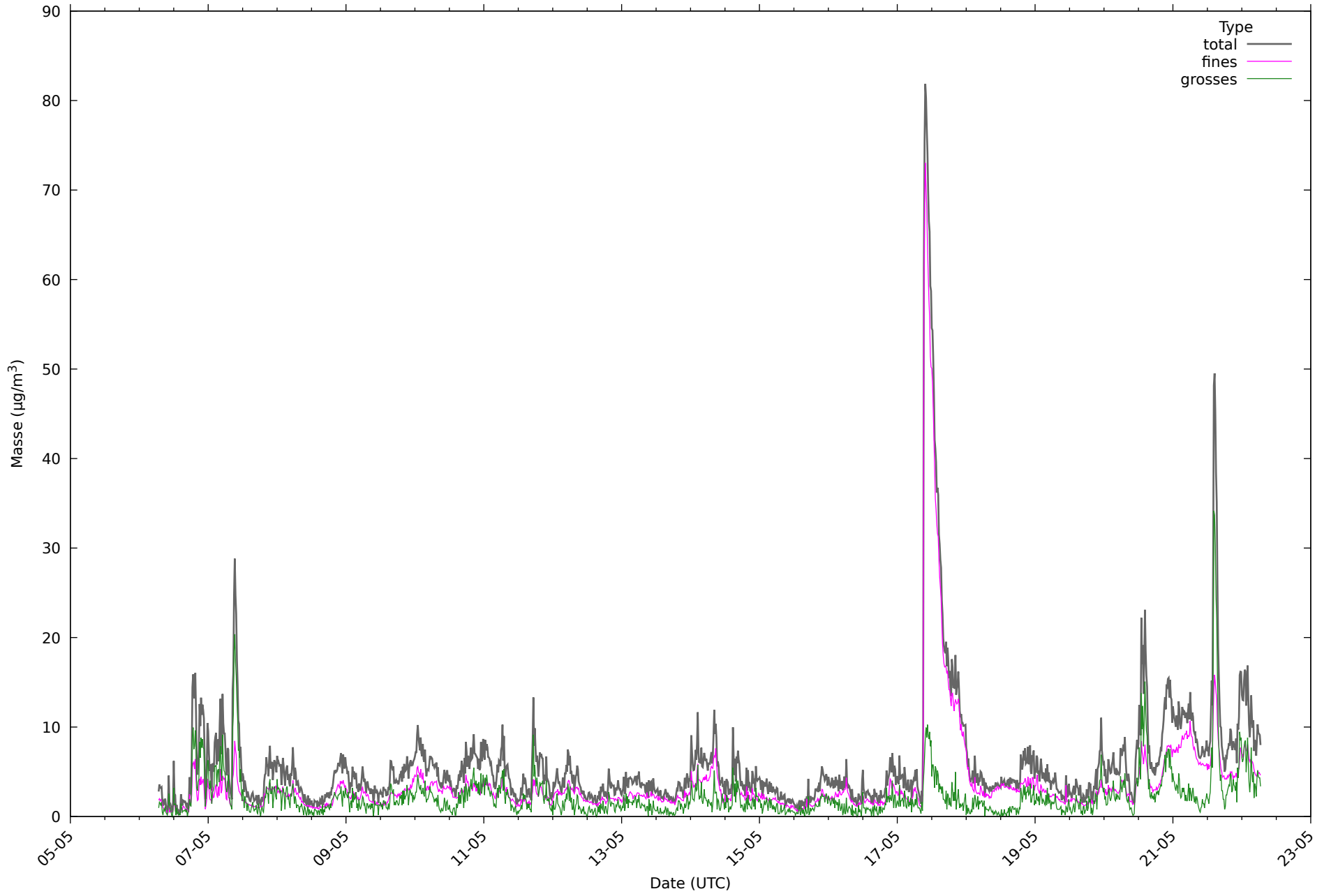
Particules sur 12 jours au 24/05/2026
