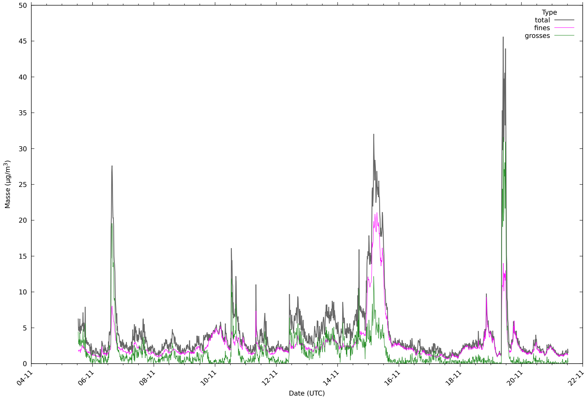
Particules sur 12 jours au 23/11/2025
