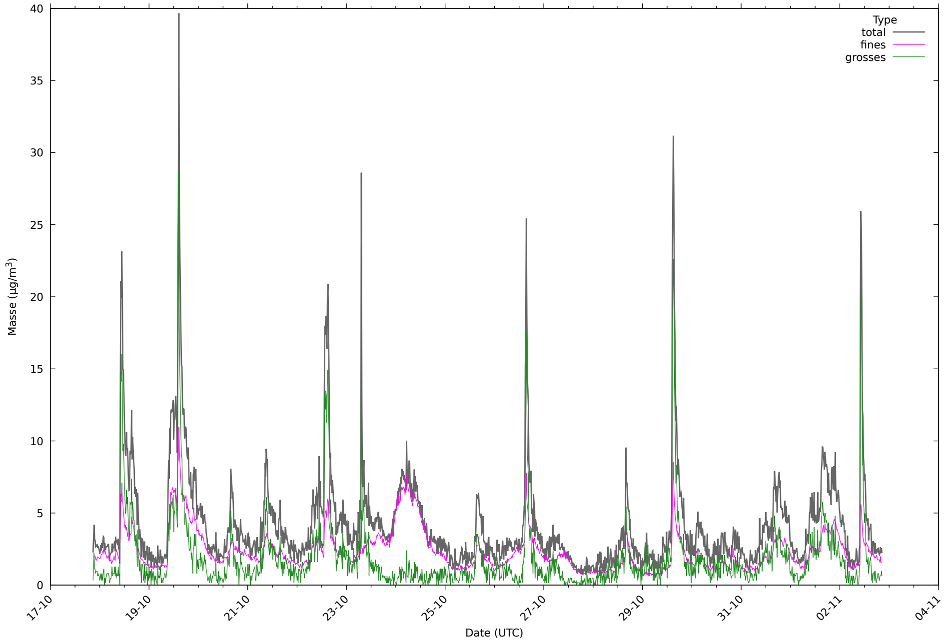
Particules sur 12 jours au 02/11/2025
