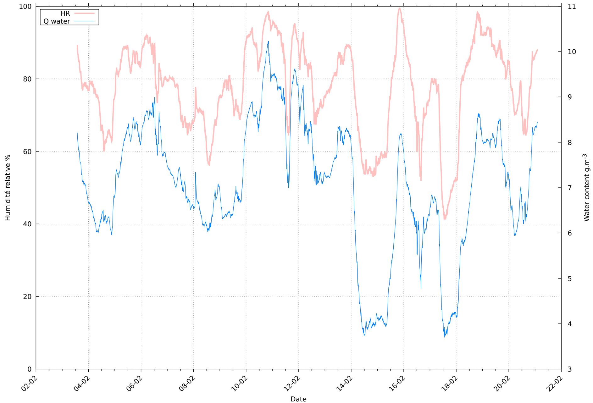
Humidité au 21/02/2026 pour RHT14
