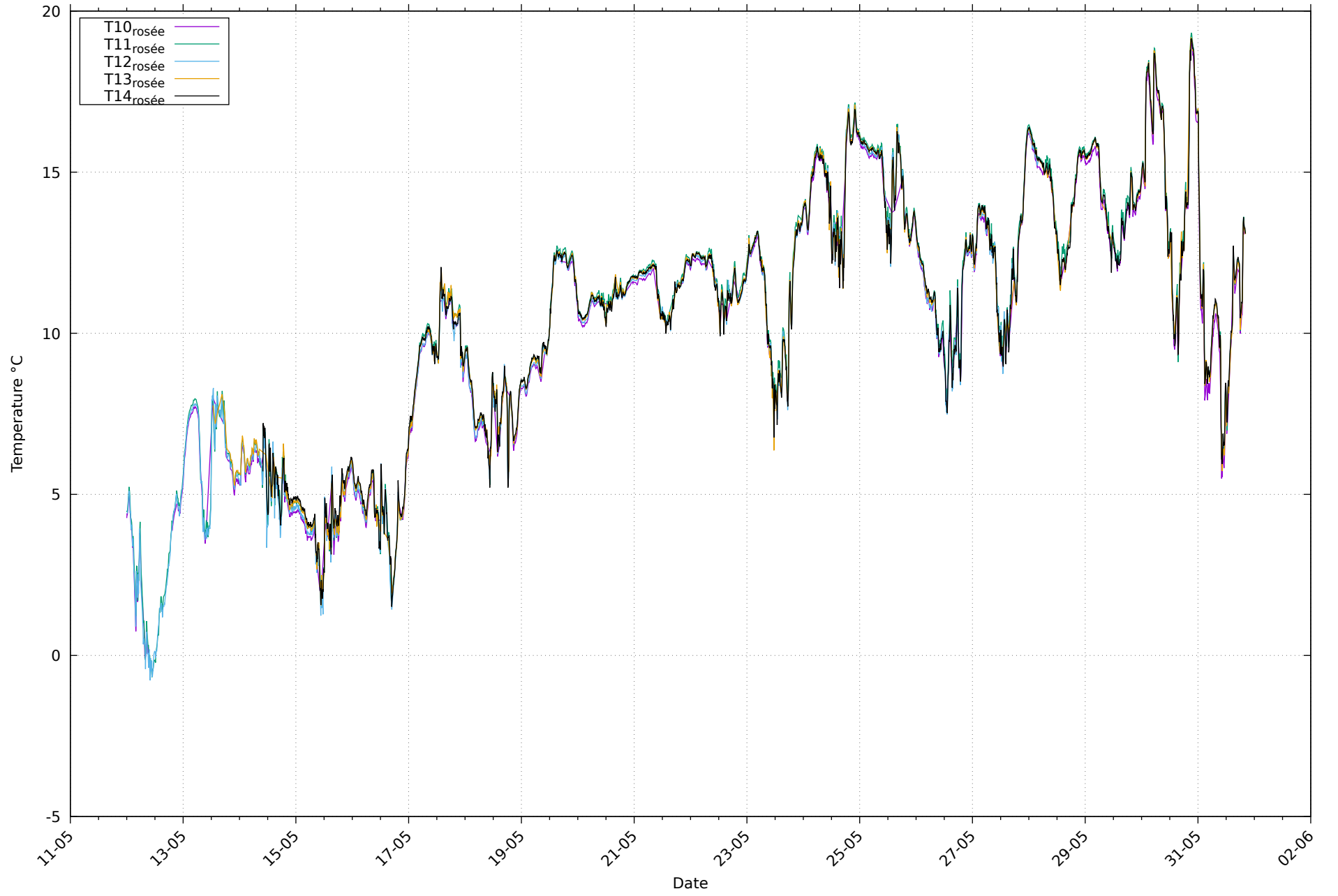
Températures de rosée au 31/05/2026
