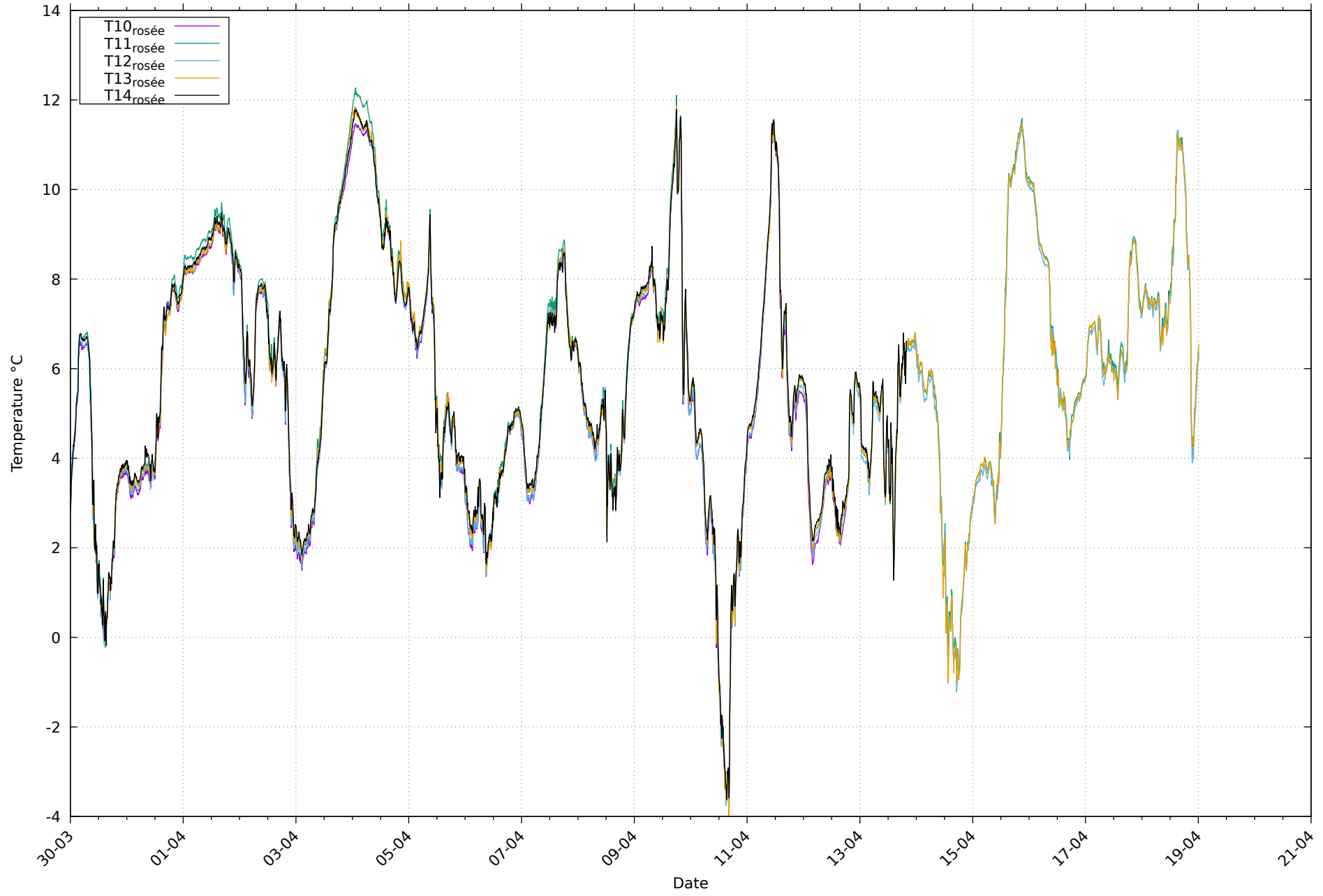
Températures de rosée au 19/04/2026
